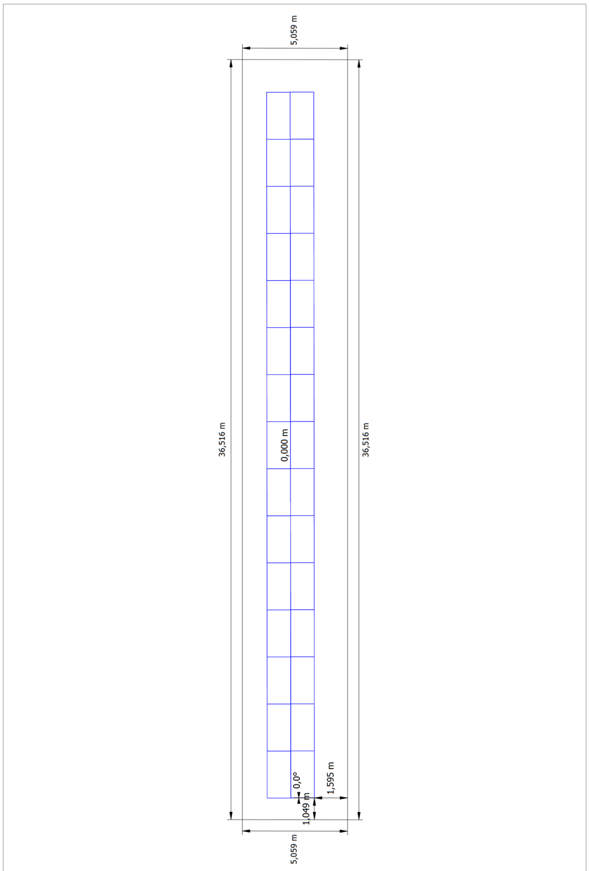
Figura: Edificio 10 - Superficie del tejado sur
