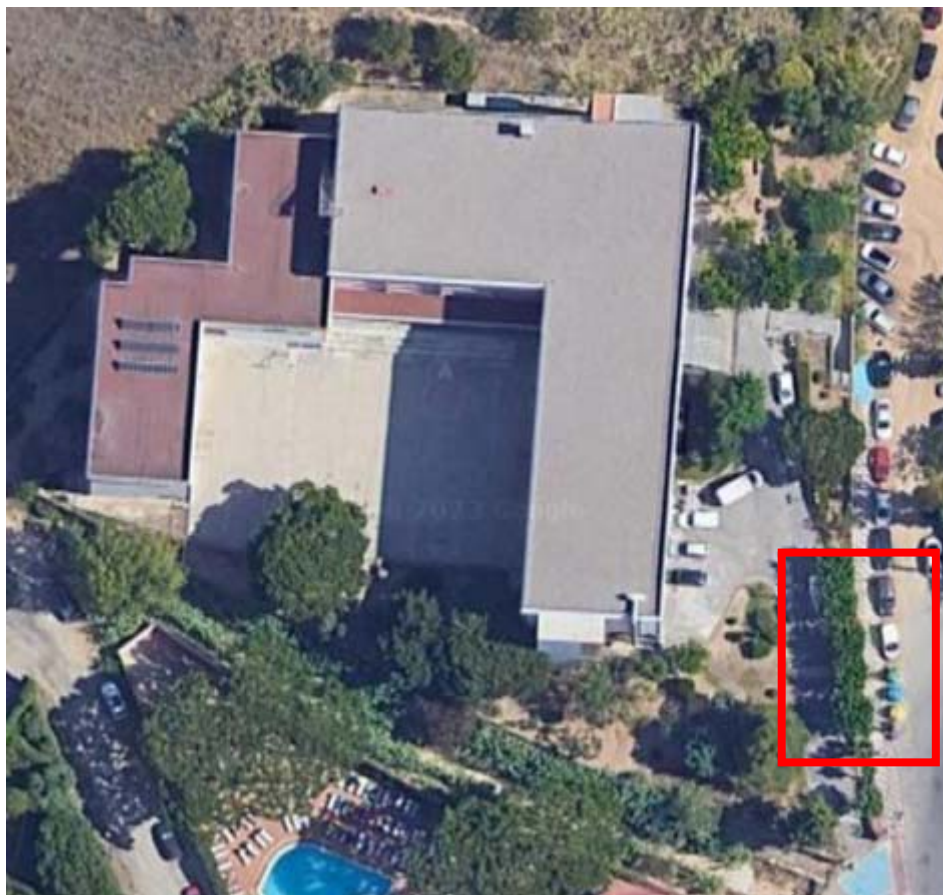
Il·lustració 10. Ubicació de la TMF-10 existent de consum i de la nova TMF-10 de generació
