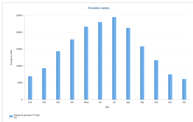
Figura 9 Producció mensual esperada. Font: PVSOL, Infraestructures.cat
