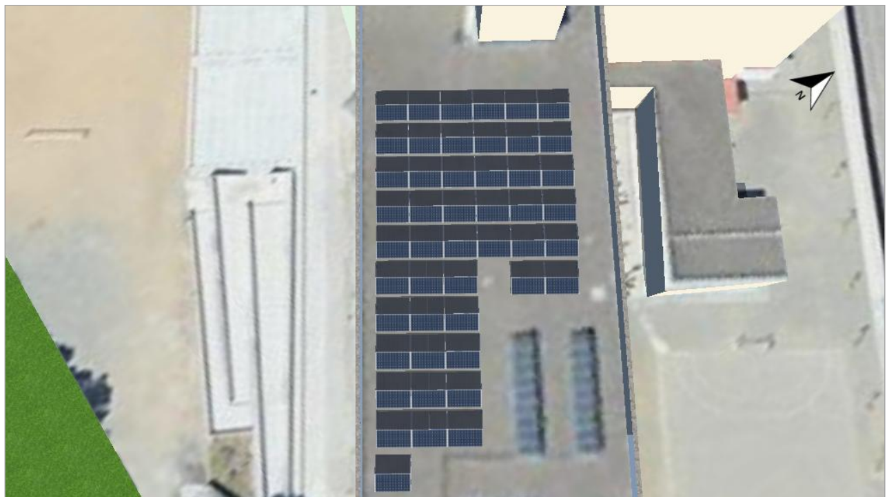
Figura: 3. Superficie fotovoltaica - Edificio a discreción 02-Superficie fotovoltaica sudeste
