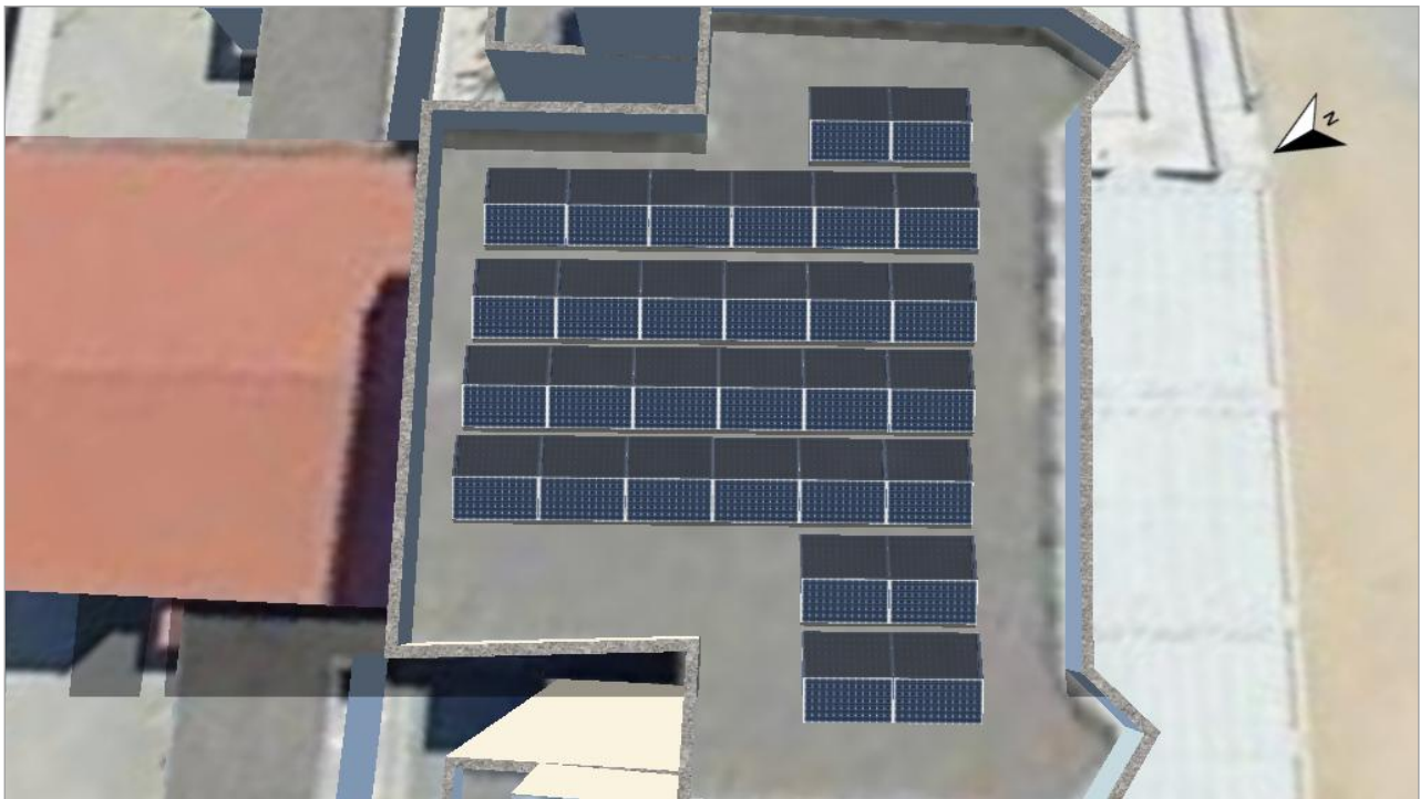
Figura: 5. Superficie fotovoltaica - Edificio a discreción 03-Superficie fotovoltaica Noroeste
