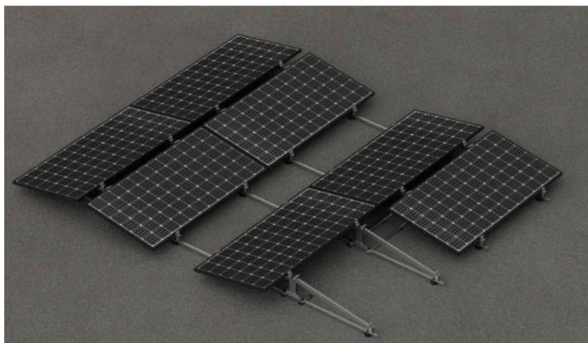
Figura 6 Estructura orientada E-O amb inclinació 10° i subjecte en costat llarg. Font: Sunfer
