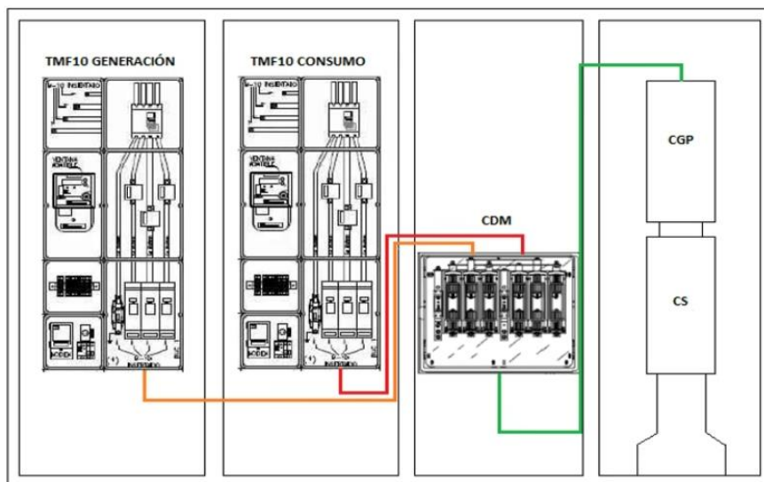
Figura 14 Esquema instal·lació per a autoconsum col·lectiu. Font: Infraestructures.cat
