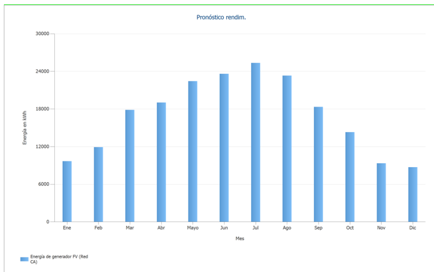
Figura 11 Gràfic de generació mensual de la instal·lació solar projectada. Font: Infraestructures.cat, PVSOL
