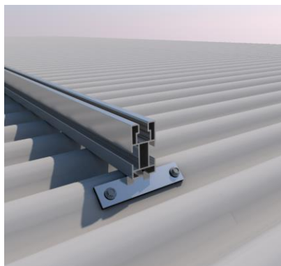
Figura 7 Solució estructural Sunfer coplanar. Font: Sunfer
