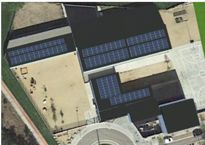
Figura 2 Simulació FV de la planta autoconsum. Font: PVSOL. Infraestructures.cat
