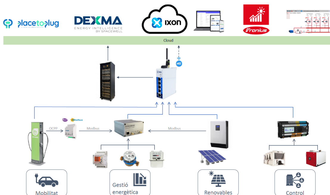
Figura 16 Esquema de connexions del sistema de comunicacions. Font: Infraestructures.cat
