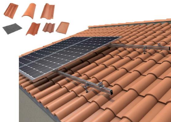
Figura 5 Solució estructural seleccionada per coberta de teula. Font: Sunfer
