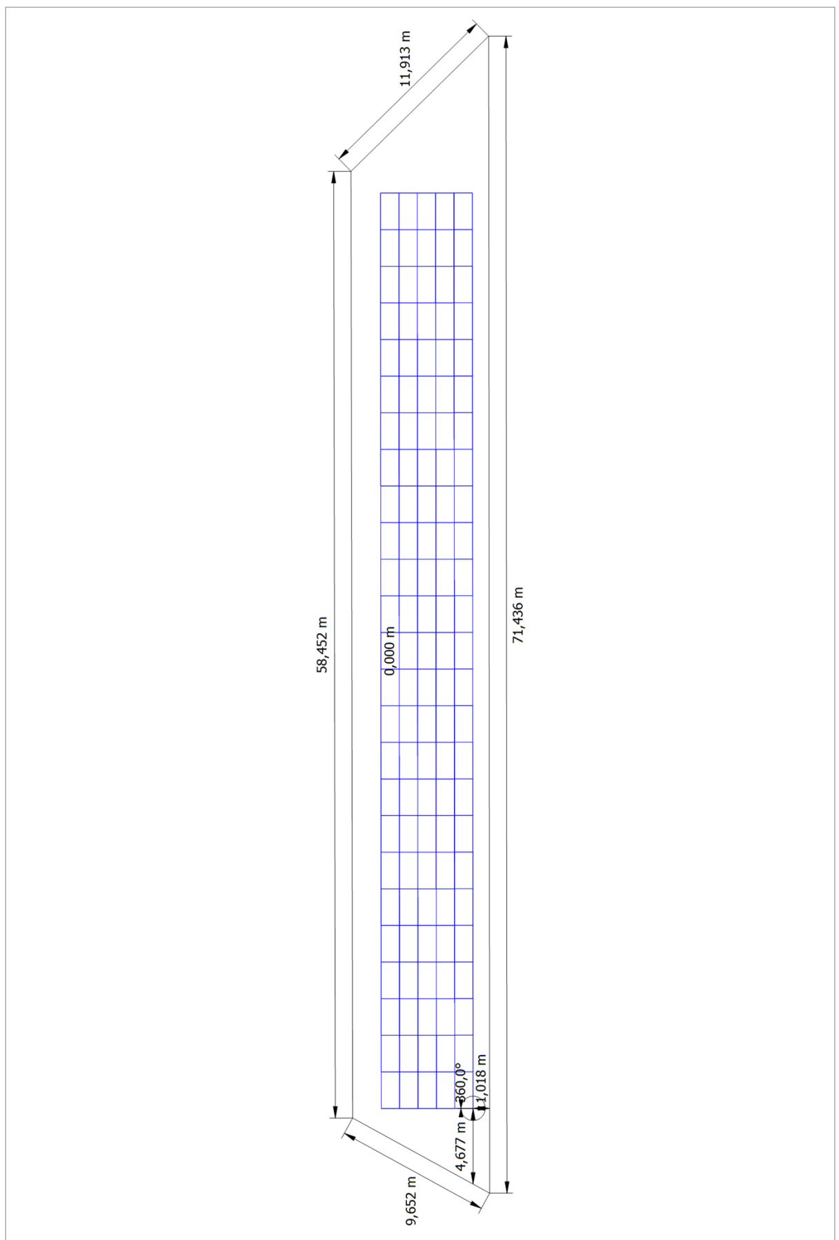
Figura: Edificio a discreción 03 - Superficie a ocupar sudeste
