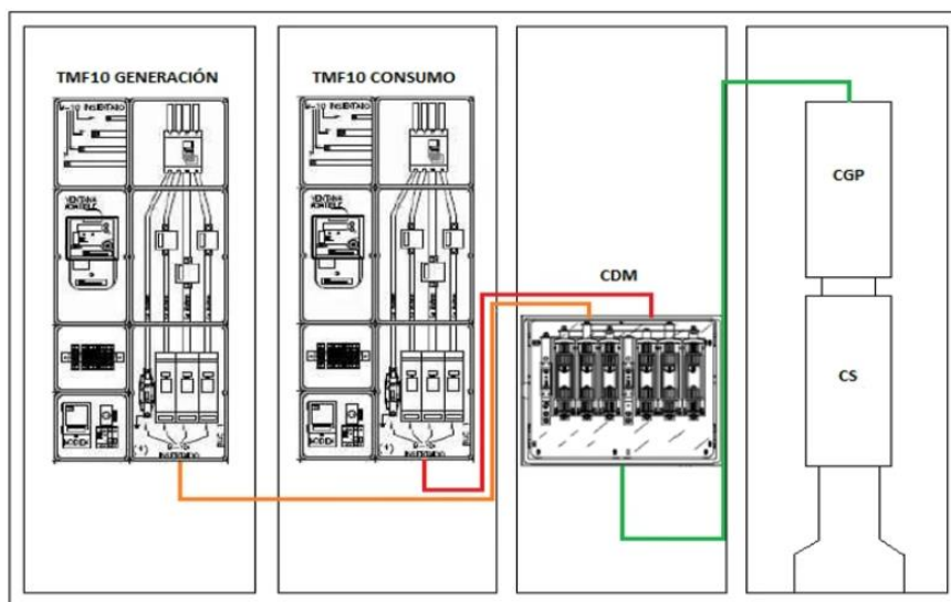
II-lustració 7. Esquema de muntatge
