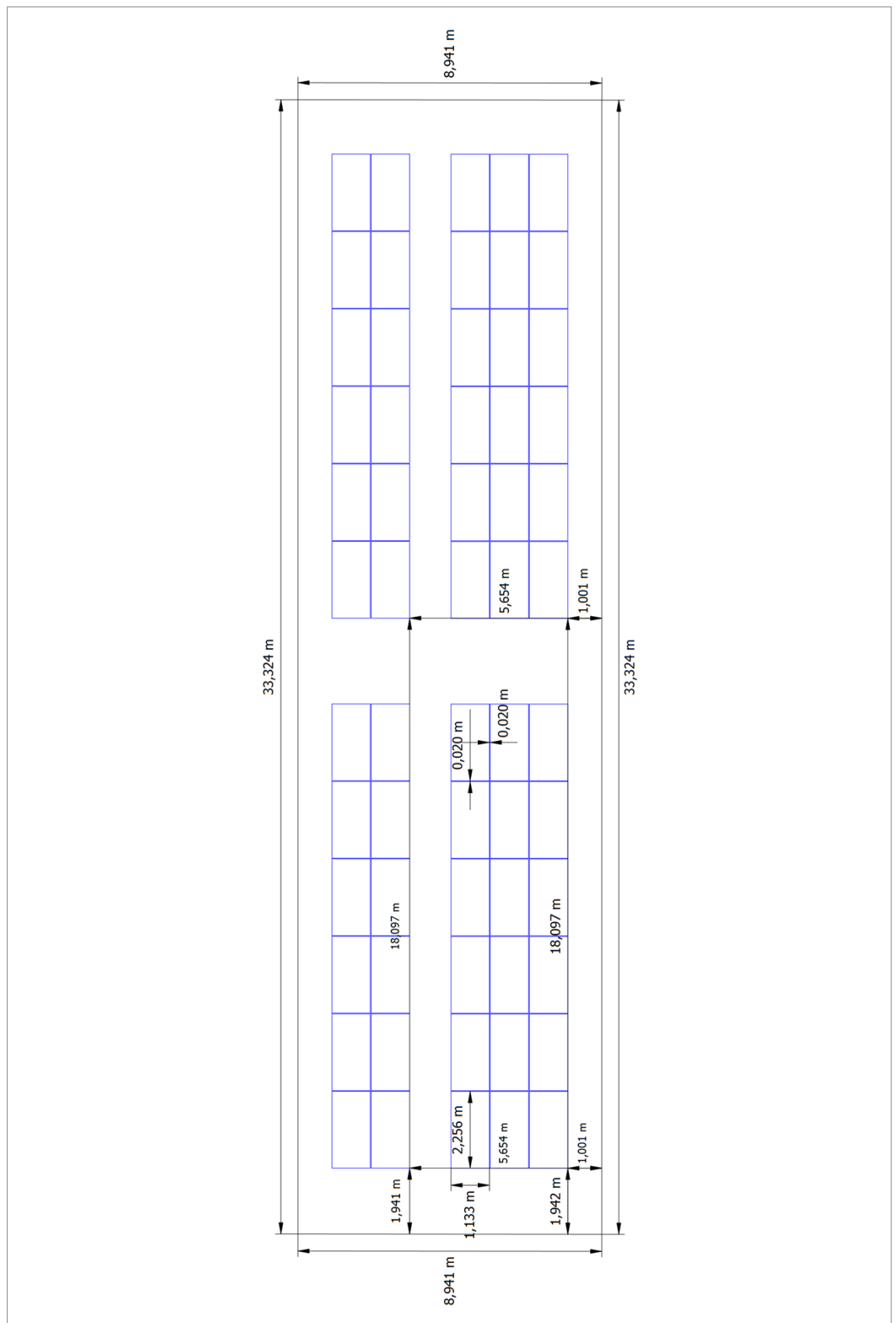
Figura: Aularis 1 - Superficie del tejado sudoeste
