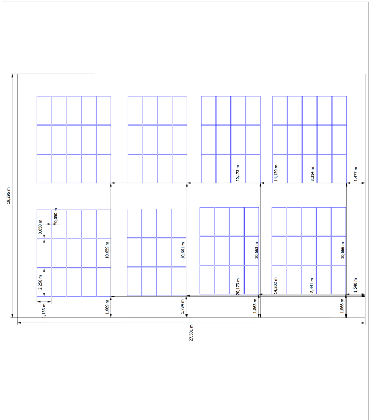
Figura: Gimnàs - Superfície del tejado sudeste
