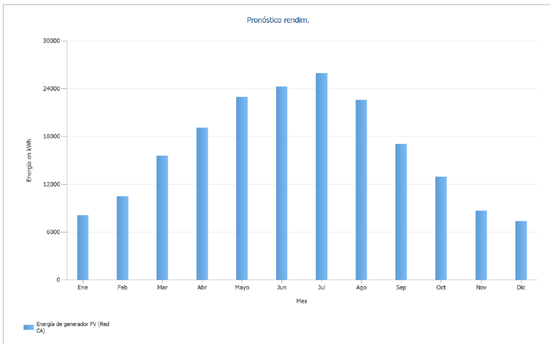
Il·lustració 6. Generació fotovoltaica anual
