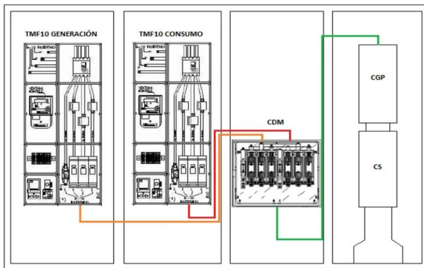
Il·lustració 8. Esquema de muntatge
