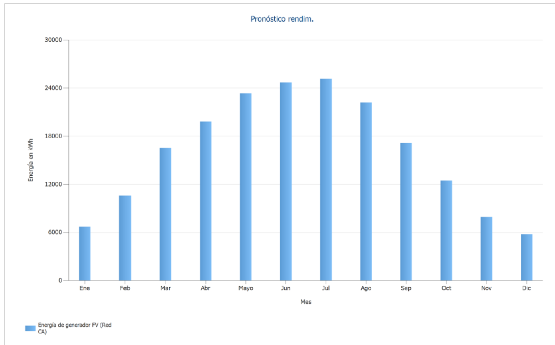
Figura: Pronóstico rendim.
