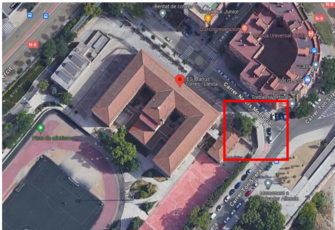
Il·lustració 8. Ubicació de les noves TMF-10 de consum i de generació
