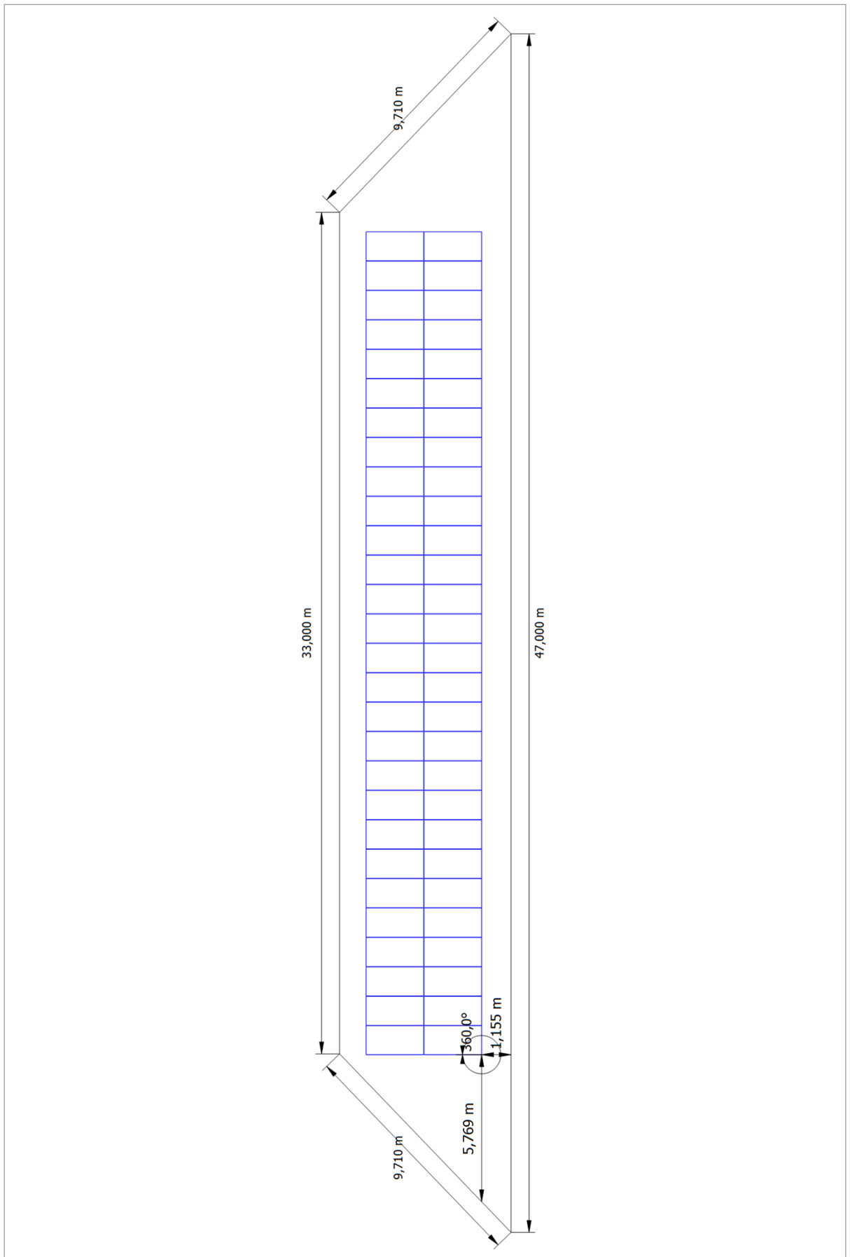
Figura: Edificio 01 - Superficie del tejado sudeste
