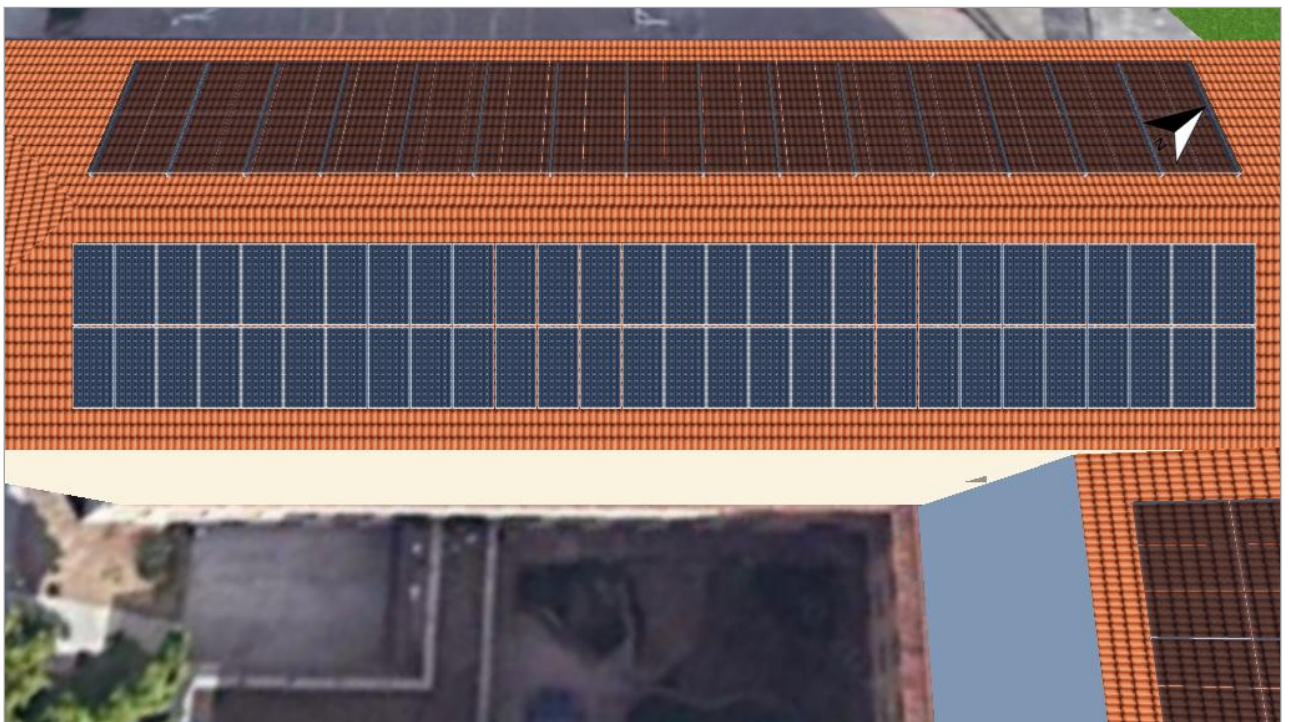
Figura: 1. Superficie fotovoltaica - Edificio 01-Superficie del tejado sudeste
