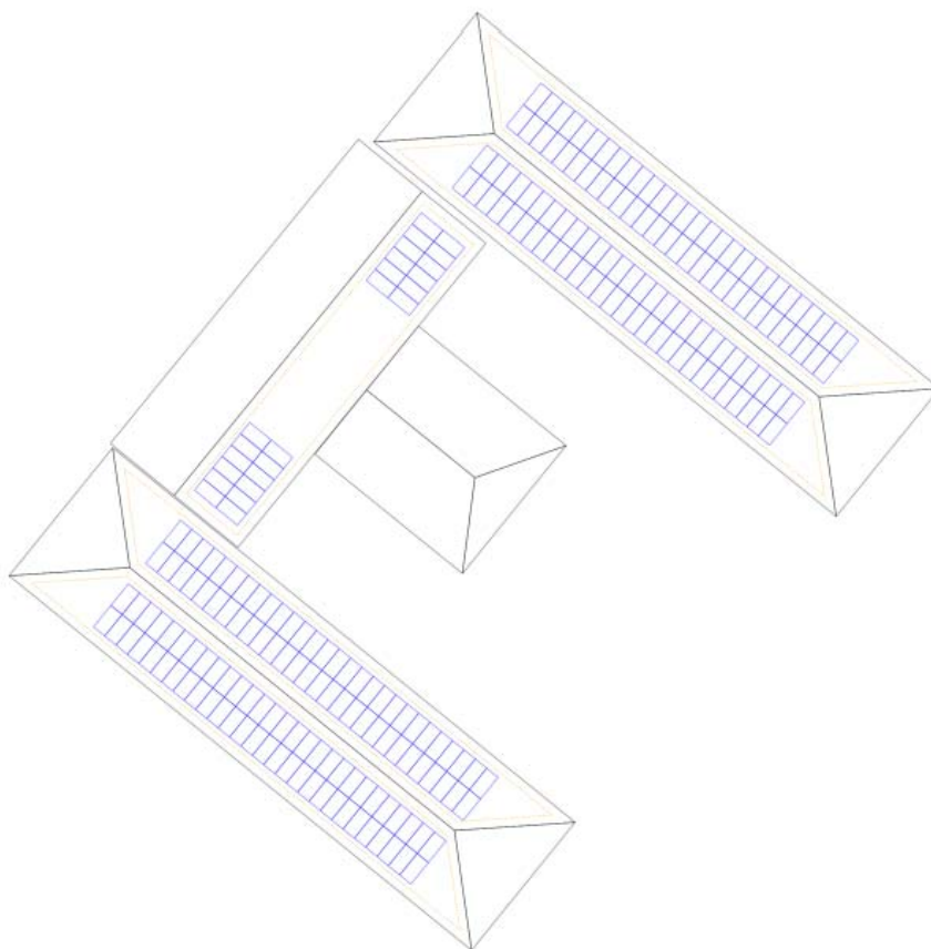
Il·lustració 2. Estudi fotovoltaic
