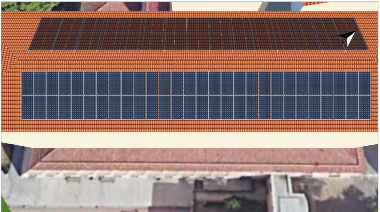
Figura: 2. Superficie fotovoltaica - Edificio 02-Superficie del tejado sudeste
