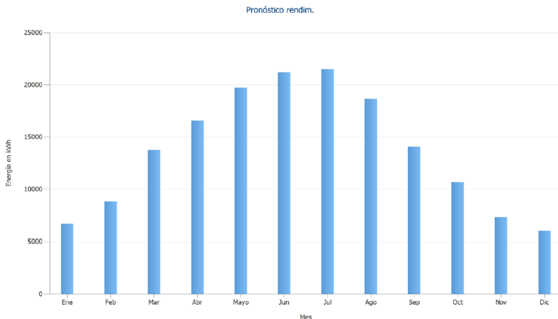
Figura 9 Producció solar i mensual esperada. Font: PVSOL, Infraestructures.cat
