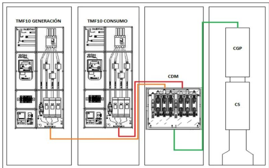
II-lustració 10. Esquema de muntatge
