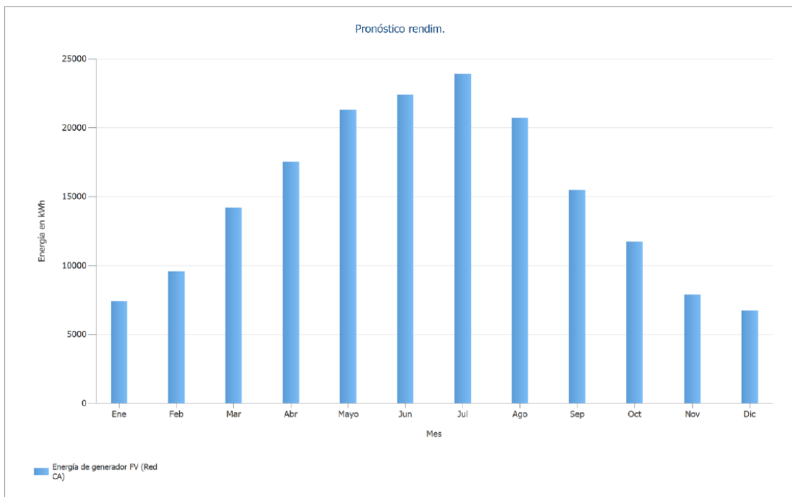
Il·lustració 8. Generació fotovoltaica anual
