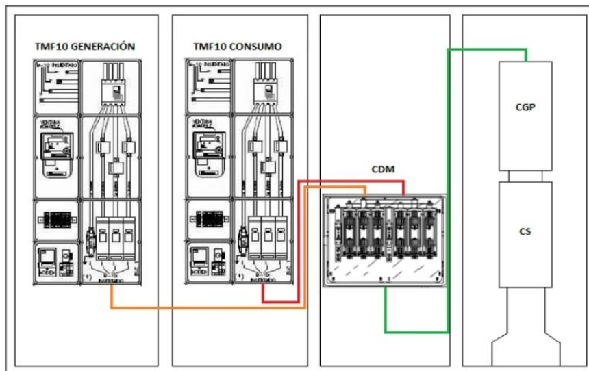
II-lustració 10. Esquema de muntatge
