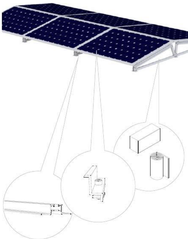
Il·lustració 6. Tipus d'estructura utilitzada
