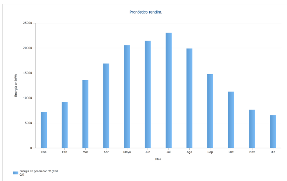
Il·lustració 8. Generació fotovoltaica anual
