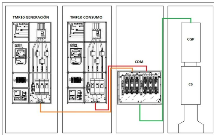
II-lustració 10. Esquema de muntatge
