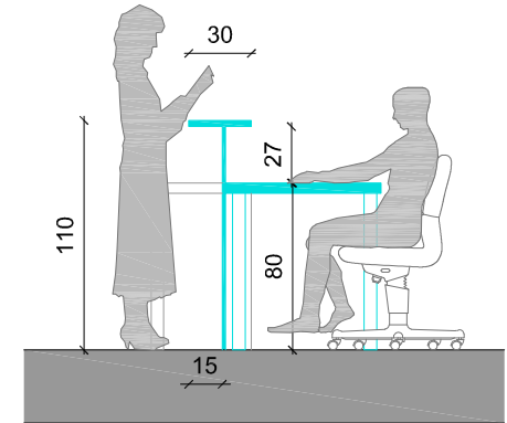
SECCIÓ B-B'
