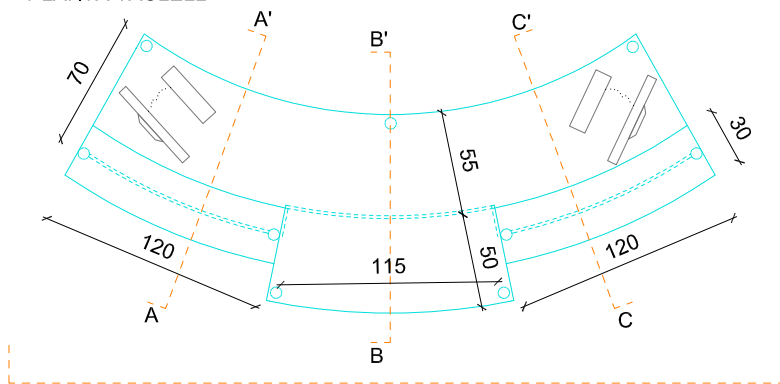
ALÇAT FRONTAL
