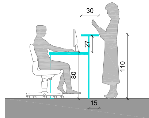
SECCIÓ C-C'
