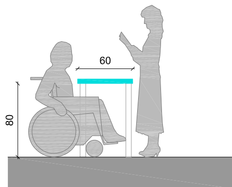
SECCIÓ A-A'
