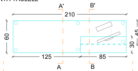
ALÇAT FRONTAL
