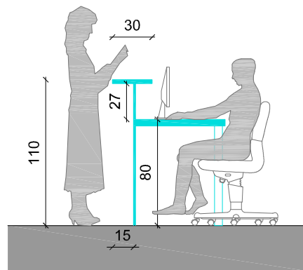
SECCIÓ A-A'
