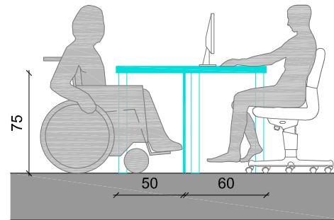
SECCIÓ A-A'
