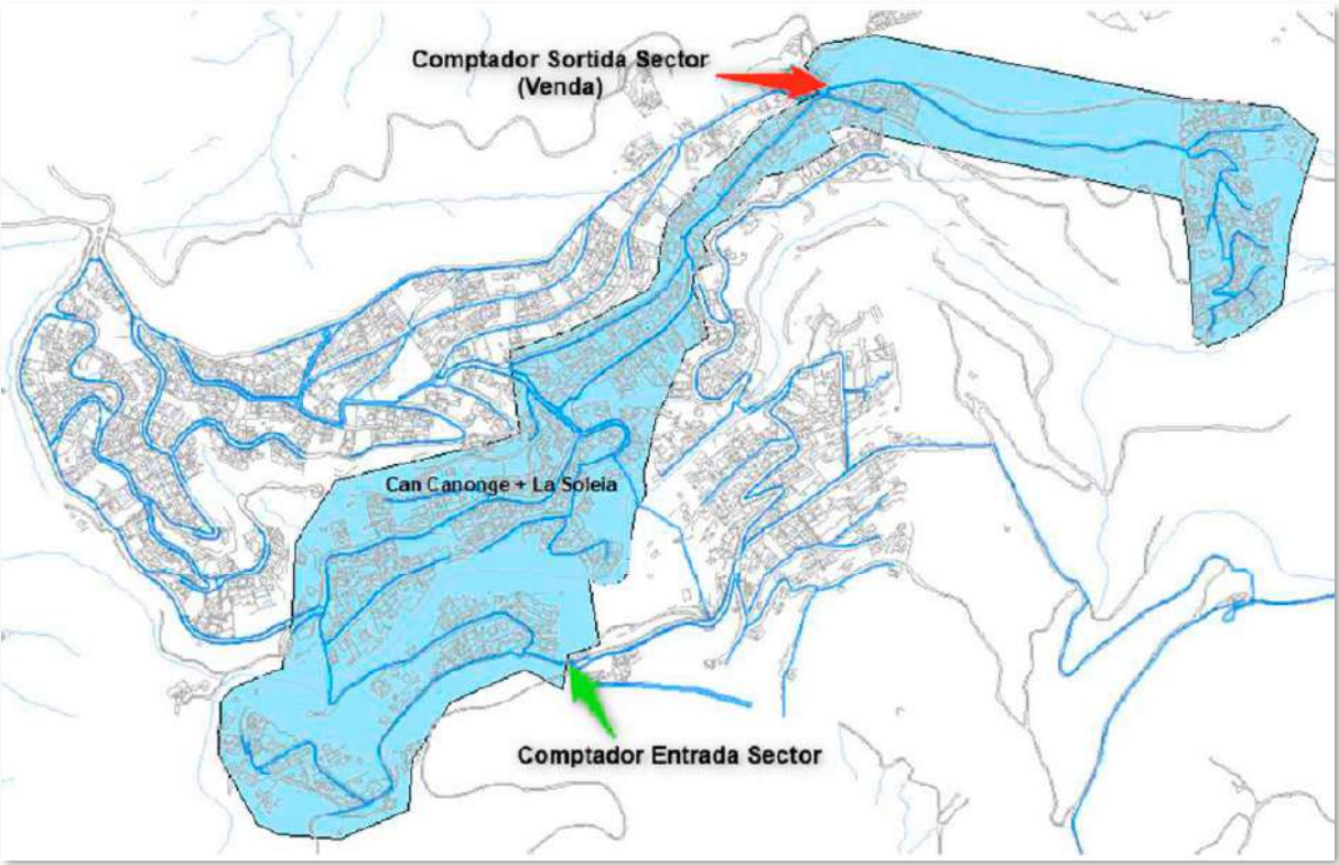
Esquema de sector d'abastament a la carretera de Corbera (Font: AGBAR)
