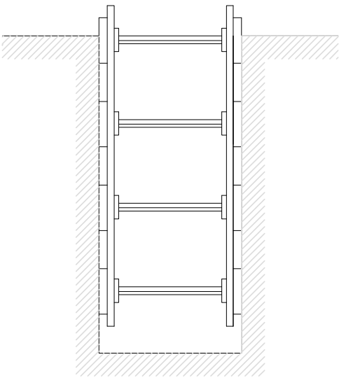
Rases amb apuntament per sobrecàrrega
