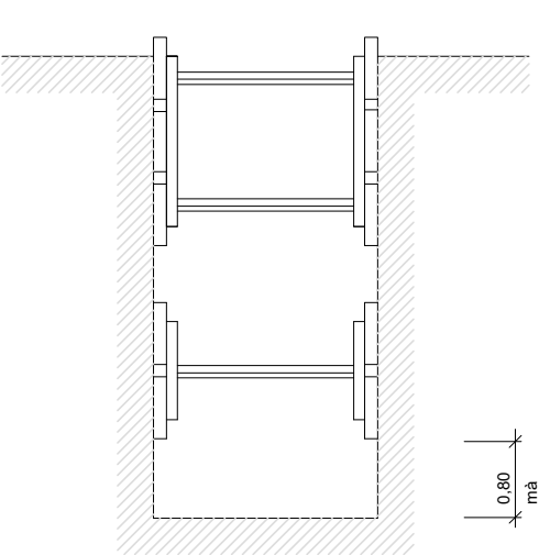
Rases amb apuntament sense sobrecàrrega
