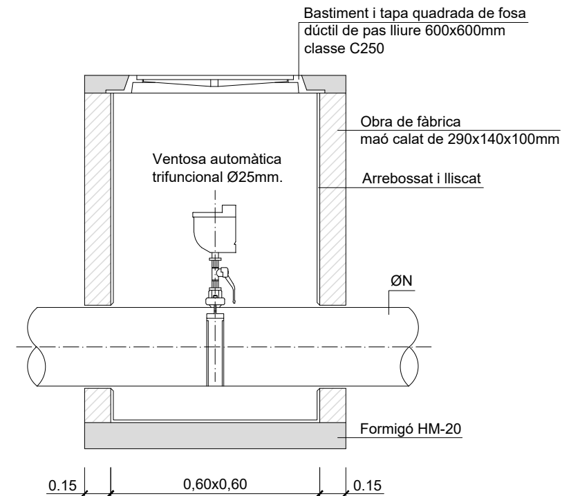
DETALL ARQUETA VÀLVULA VENTOSA I VÀLVULA DE COMPORTA DN≥150
