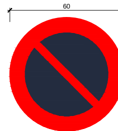
R-308. Estacionament prohibit. esc.: 1/10 (cotes en cm)
