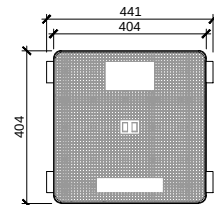
PLANTA MARC i TAPA 40x40cm Esc.: 1/10 (cotes en cm)
