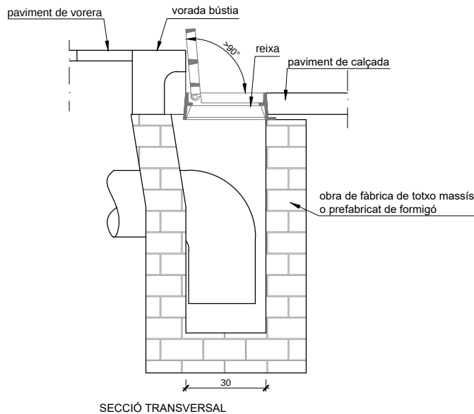
SECCIÓ TRANSVERSAL
