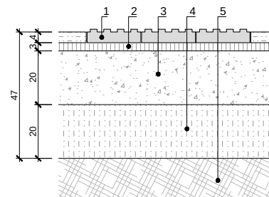
DETALL PAVIMENT PTI BOTONERA DE PECES DE 20x20x10cm Esc.: 1/10 (cotes en cm)
