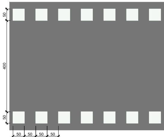
M-4.4 Pas de vianants amb semàfor. esc.: 1/50 (cotes en cm)
