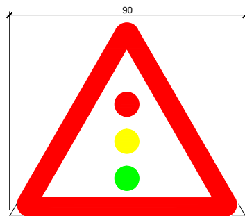
P-3 Perill. Semàfor. esc.: 1/10 (cotes en cm)
