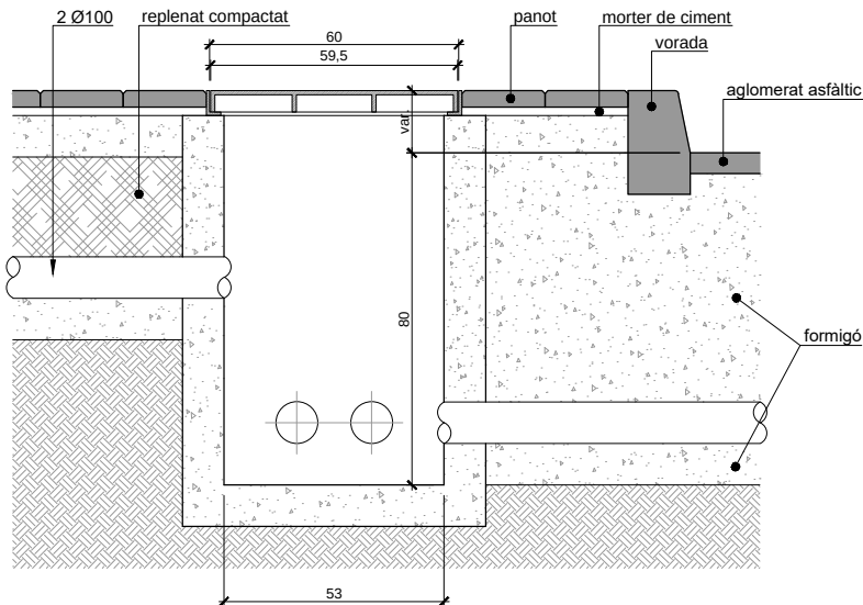
ARQUETA 60X60cm Esc.: 1/10 (cotes en cm)
