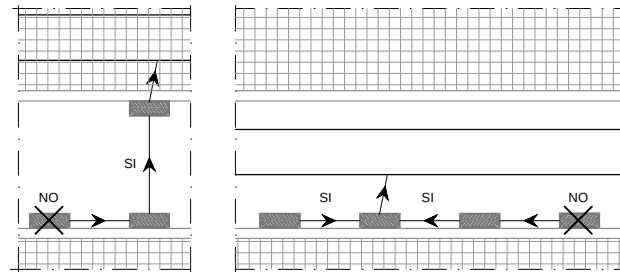
DISPOSICIONS DE CONNEXIONS D'EMBORNALS ADMESES Esc.: s/e
