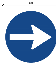
R-400a Sentit obligatori. A la dreta. esc.: 1/10 (cotes en cm)
