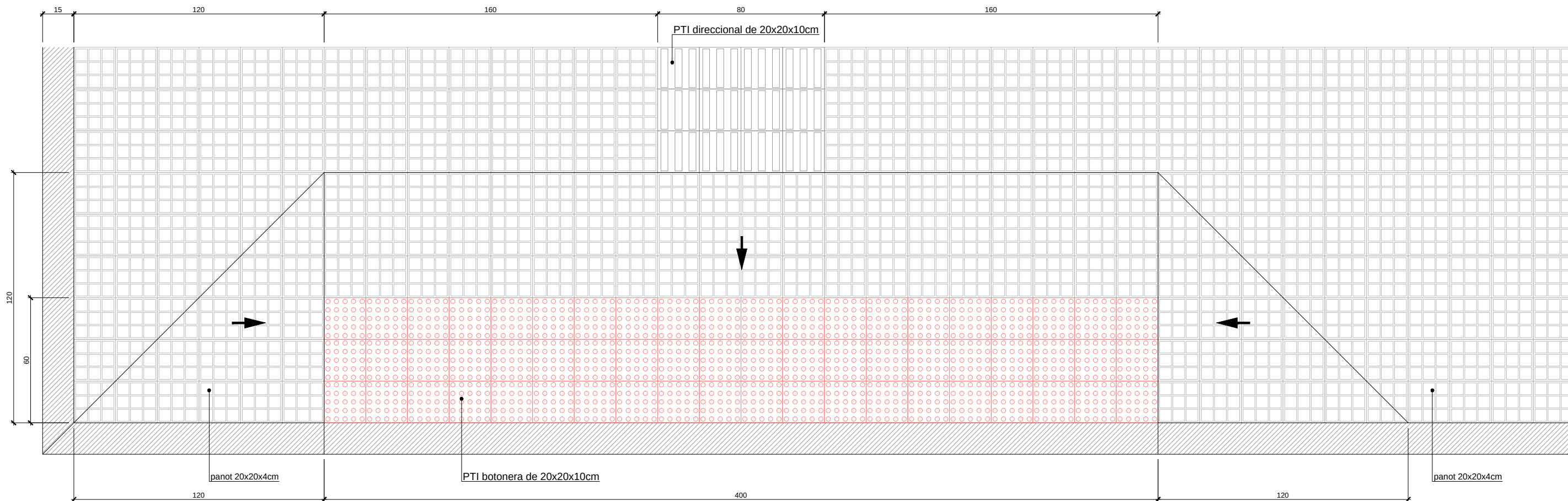
DETALL PAS DE VIANANTS Esc.: 1/10 (cotes en cm)
