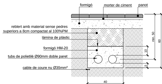
CANALITZACIÓ A VORERA. 2 TUBS Esc.: 1/10 (cotes en cm)
