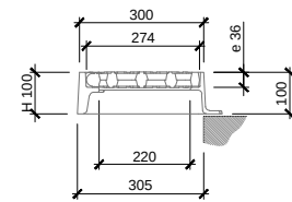
SECCIÓ TRANSVERSAL TANCADA
