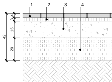
DETALL PAVIMENT DE PANOT DE 20x20x4cm Esc.: 1/10 (cotes en cm)
