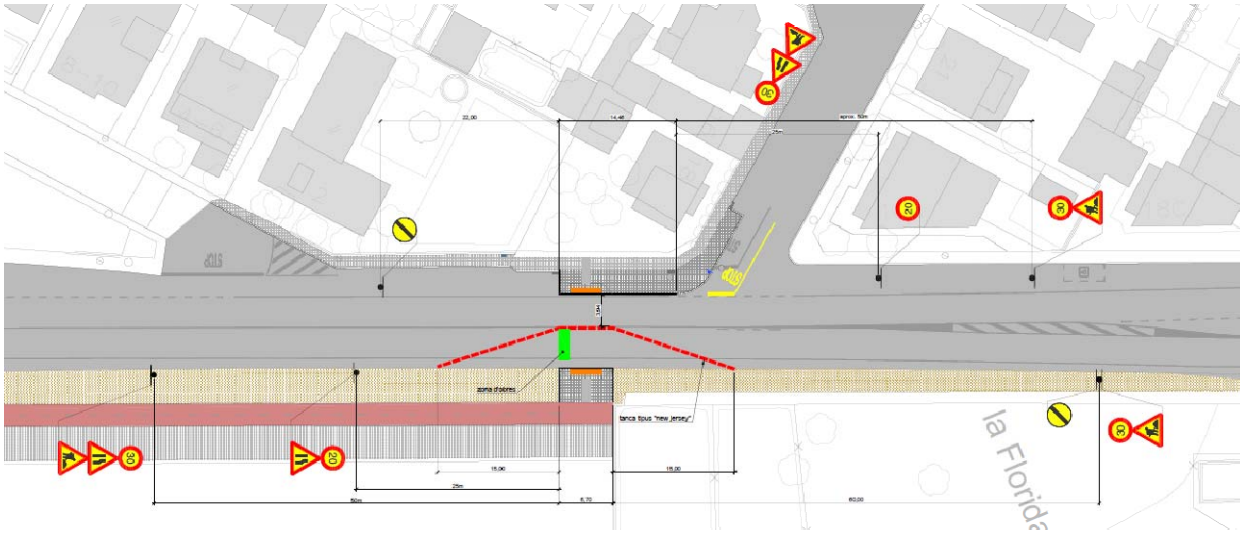
tancaments: creuament de calçada
