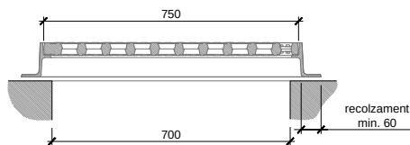
SECCIÓ LONGITUDINAL
