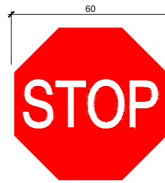
R-2 Detenció obligatòria. STOP. esc.: 1/10 (cotes en cm)
