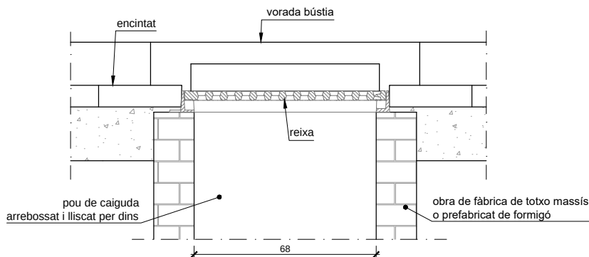
SECCIÓ LONGITUDINAL
