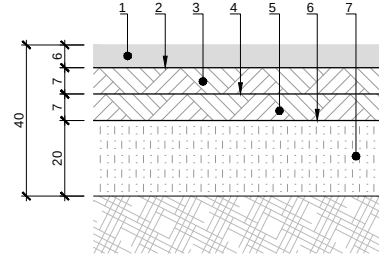
DETALL REPOSICIÓ PAVIMENT BITUMINÓS Esc.: 1/10 (cotes en cm)
