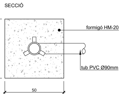
PLANTA FONAMENTACIÓ BÀCUL DE SEMÀFOR Esc.: 1/10 (cotes en cm)
