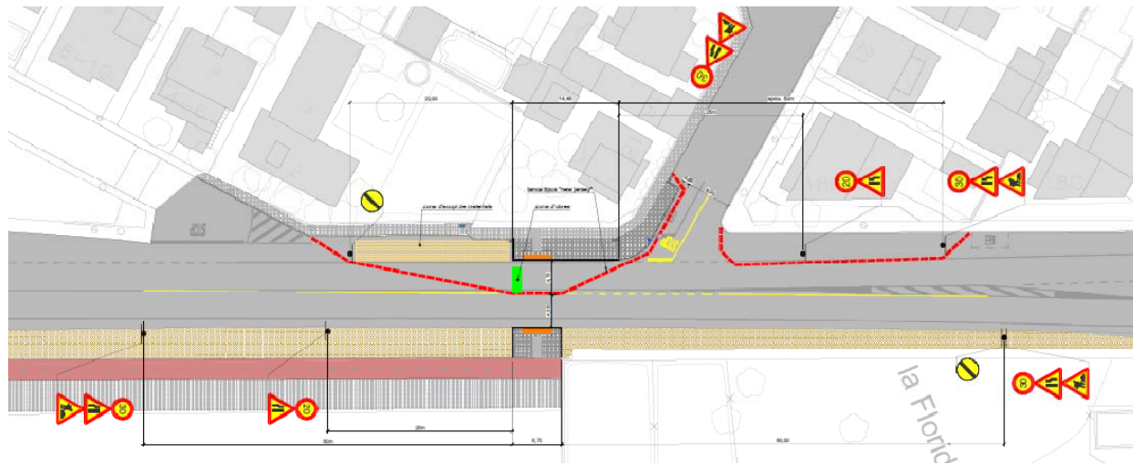
tancaments: creuament de calçada
