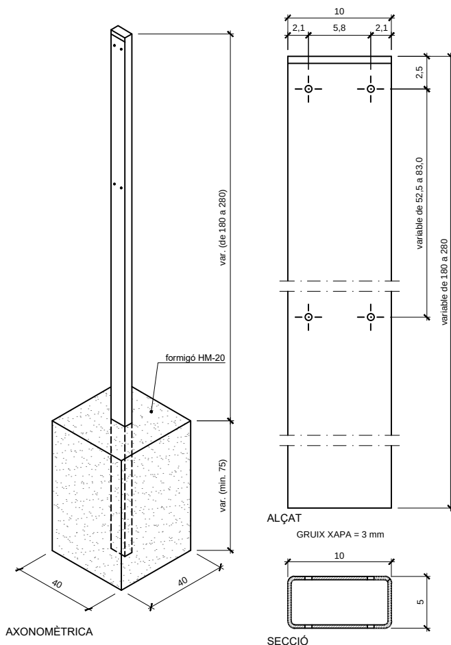
SUPORT PER A SENYALITZACIÓ VERTICAL
