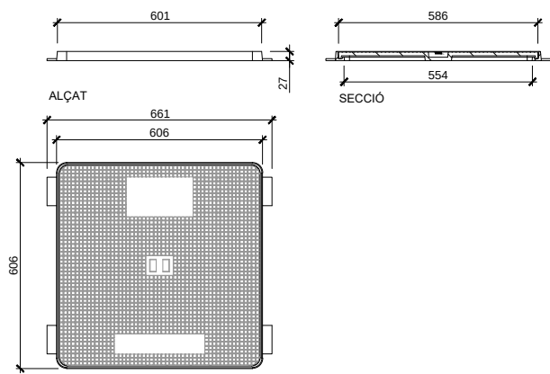
PLANTA MARC i TAPA 60x60cm Esc.: 1/10 (cotes en cm)
