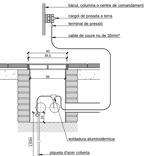
PRESA DE TERRA Esc.: s/e (cotes en cm)
