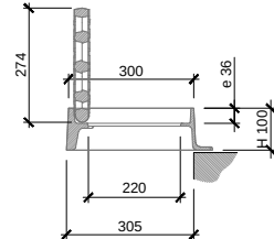
SECCIÓ TRANSVERSAL OBERTA
