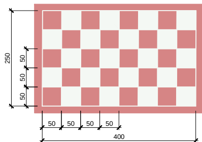
Carril Bici. ESCAQUER 50x50cm (400x250cm). esc.: 1/50
