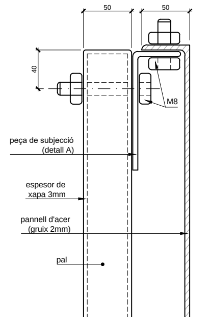
DETALL UNIÓ SUPERIOR SUPORT - SENYAL Esc.: 1/2 (cotes en mm)
