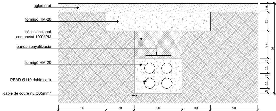
REPOSICIÓ EN CREUAMENTS DE CALÇADA. 4 TUBS Esc.: 1/10 (cotes en cm)
