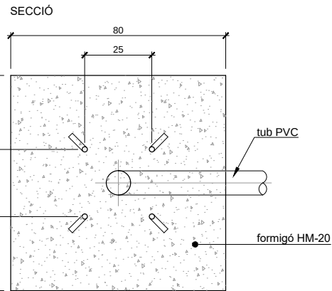
PLANTA FONAMENTACIÓ BÀCUL DE SEMÀFOR Esc.: 1/10 (cotes en cm)
