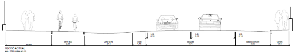
Secció existent
