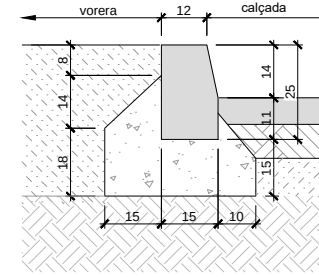
VORADA PREFABRICADA DE FORMIGÓ TIPUS T2 DE 100x15x25cm Esc.: 1/10 (cotes en cm)
