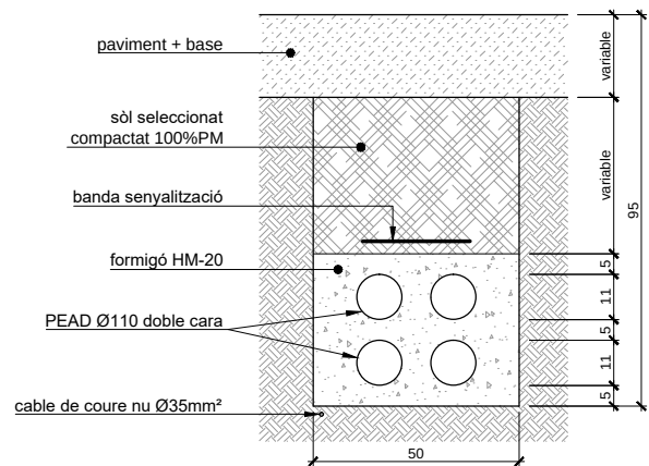
CANALITZACIÓ EN CALÇADA. 2 TUBS Esc.: 1/10 (cotes en cm)
