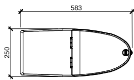
PLANTA PROJECTOR h=6m esc.: 1/10 (cotes en mm)
