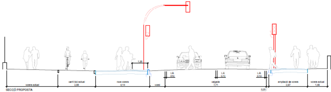
Secció proposta
