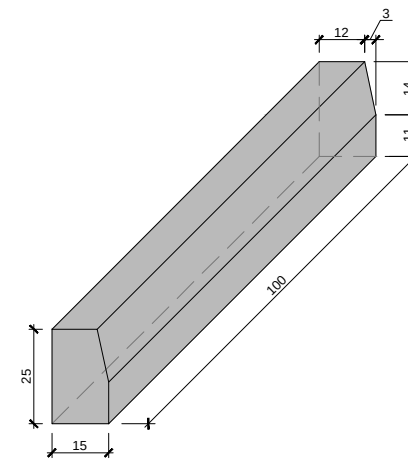
PERSPECTIVA VORADA TIPUS T2 Esc.: 1/10 (cotes en cm)
