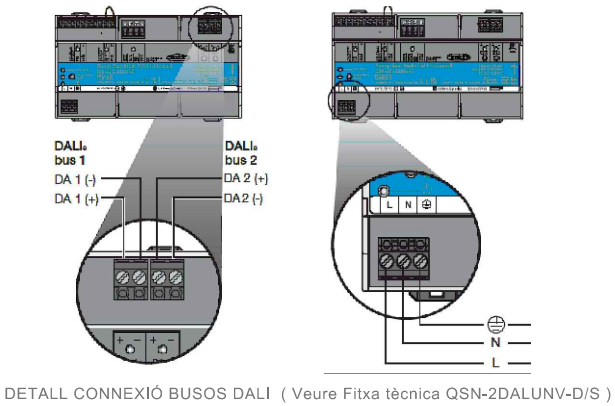
DETALL CONNEXIÓ BUSOS DALI ( Veure Fitxa tècnica QSN-2DALUNV-D/S )
