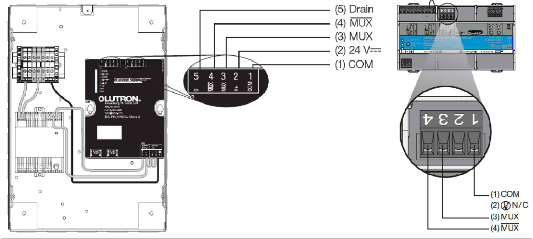
DETALL CONNEXIÓ CABLE LINK QS ( Veure Fitxa tècnica QP3-1P0CSE-230 i fitxa tècnica QSN-2DALUNV-D/S )
