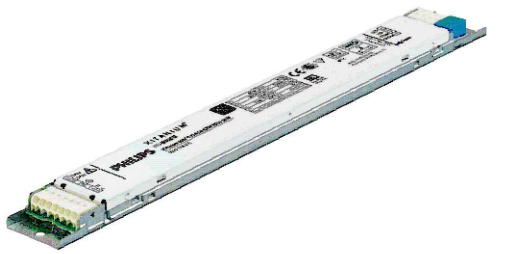
2 UNITATS EQUIPS ALIMENTACIÓ PER LLUMINÀRIA Xitanium 35W 0.08-0.35A 220V TD11 230 Certificació DALI-2 ( 102, 251, 252 i 253 )
