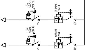
NOUS CIRCUITS QUADRE 1:2 SAI
