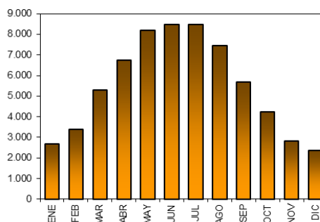
Figura 3. Producció obtinguda a partir de les dades de radiació solar de l'Atles de Catalunya.
