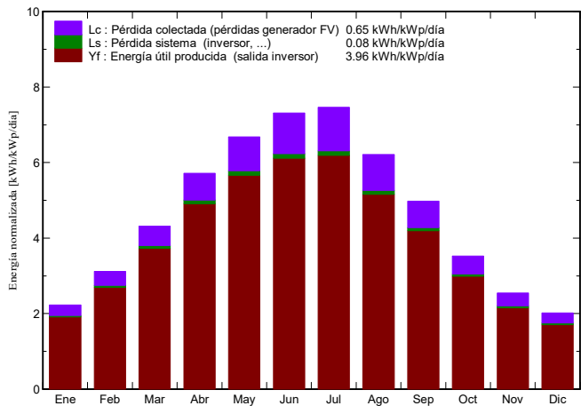
Producciones normalizadas (por kWp instalado): Potencia nominal 49.0 kWp
