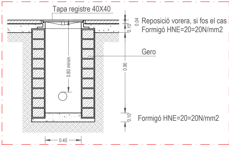
DETALL ARQUETA DE BAIXA TENSIÓ e; 1/25
