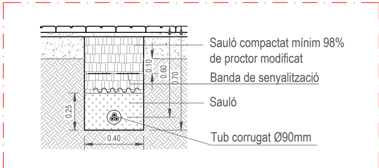
DETALL RASA EN VORERA - BAIXA TENSIÓ e; 1/25
