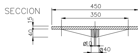
DETALL TAPA D'ARQUETA DE REIGSTRE
