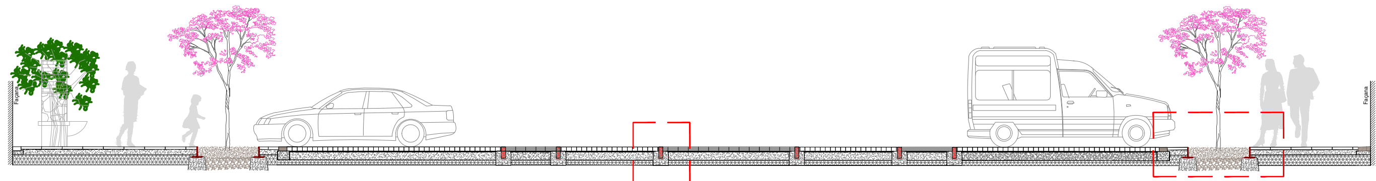
DETALL CENTRE-PLAÇA E=1:25
