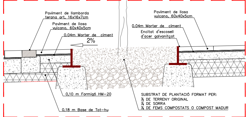
DETALL TROBADA VORERA-PLAÇA E=1:25
