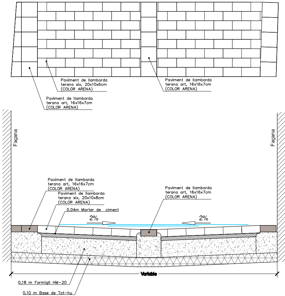
SECCIÓ BB' E=1:25
