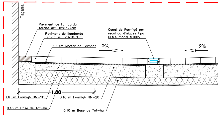
SECCIÓ DD' E=1:75
