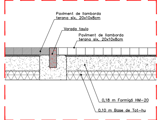
DETALL CENTRE-PLAÇA E=1:25
