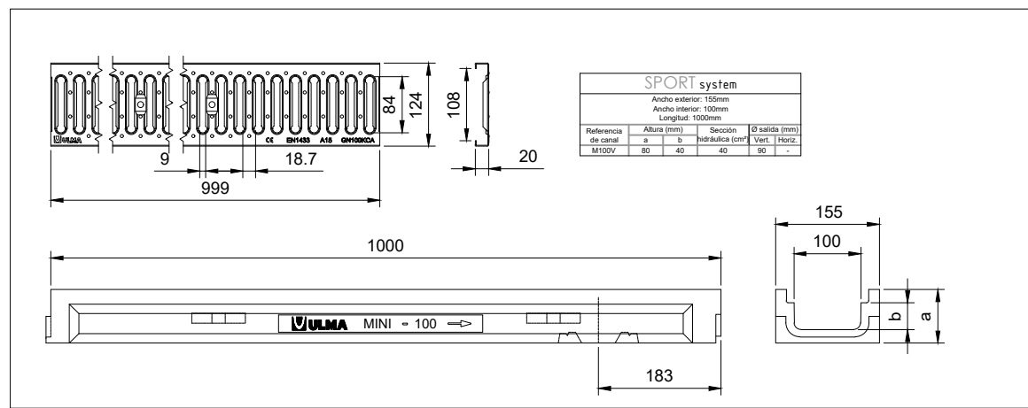
DETALL DRENATGE I REIXA E=1:10
