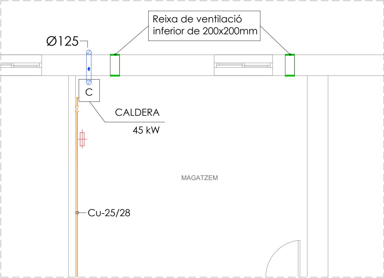
SALA DE CALDERES - 1/50
