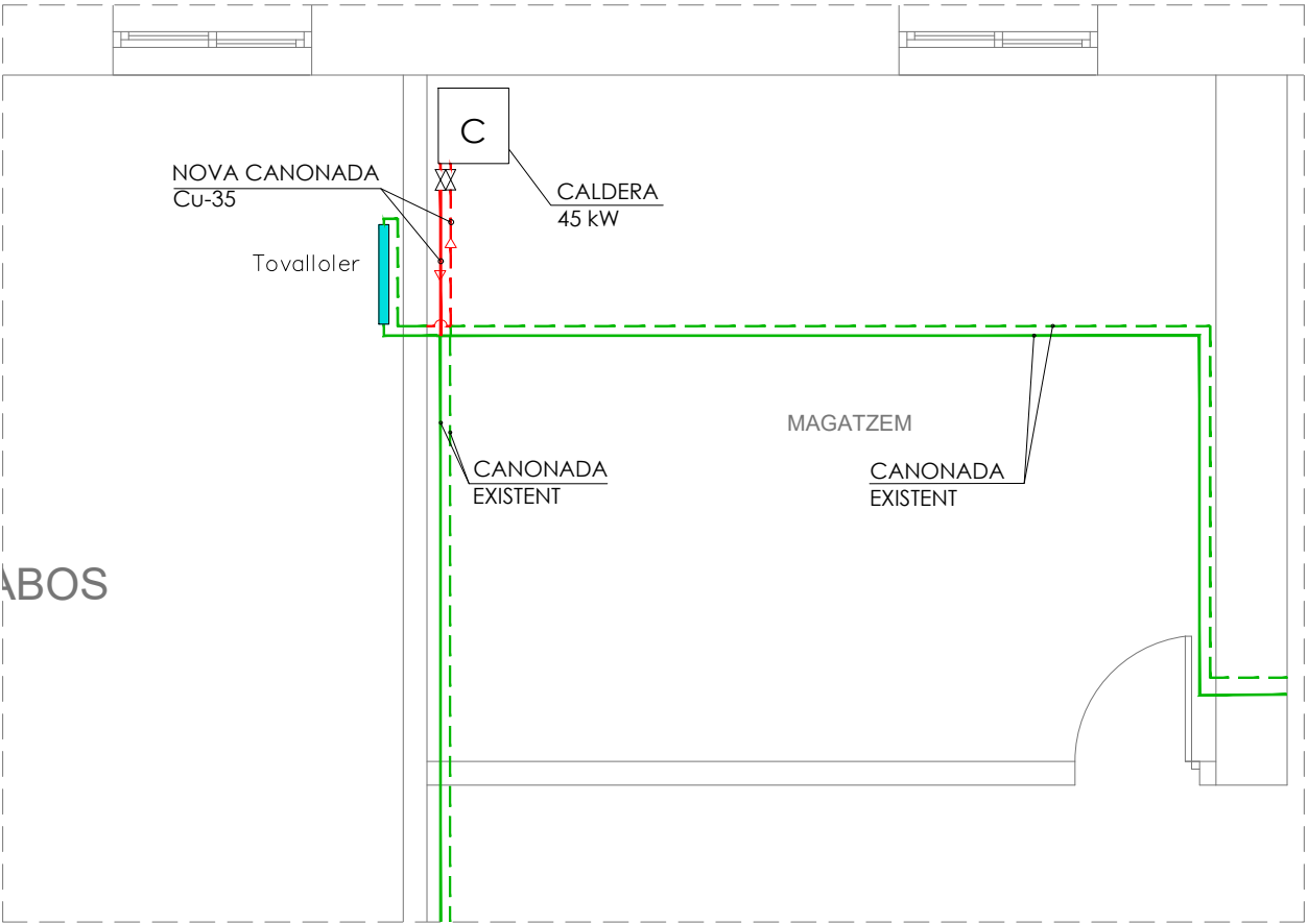
SALA DE CALDERES CIRCUI T HIDRÀULIC - 1/50
