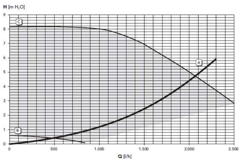
fig. 27 - Pérdidas de carga/altura manométrica circulador
