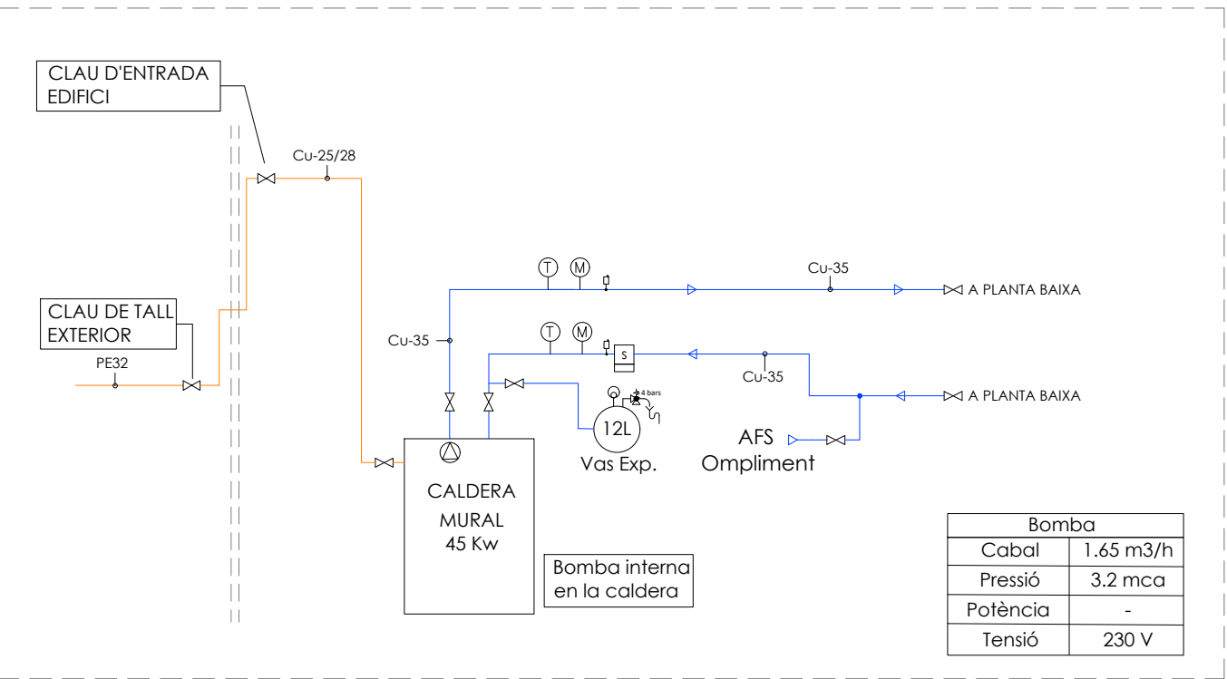
ESQUEMA SALA DE CALDERES
