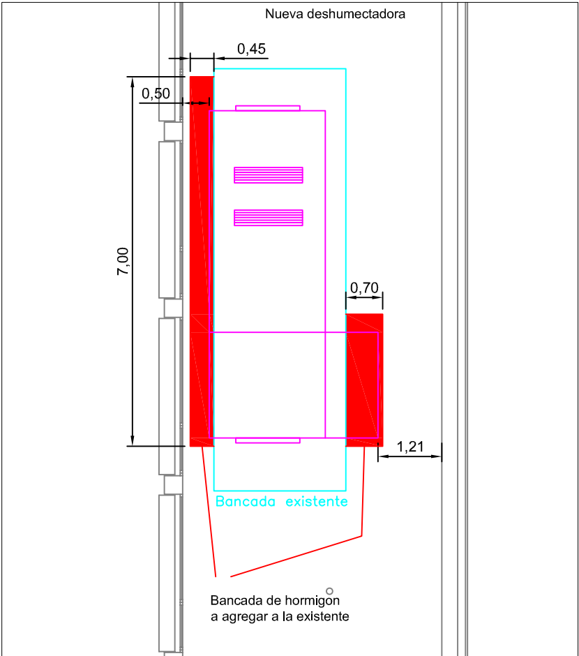
Reforma bancada existente
