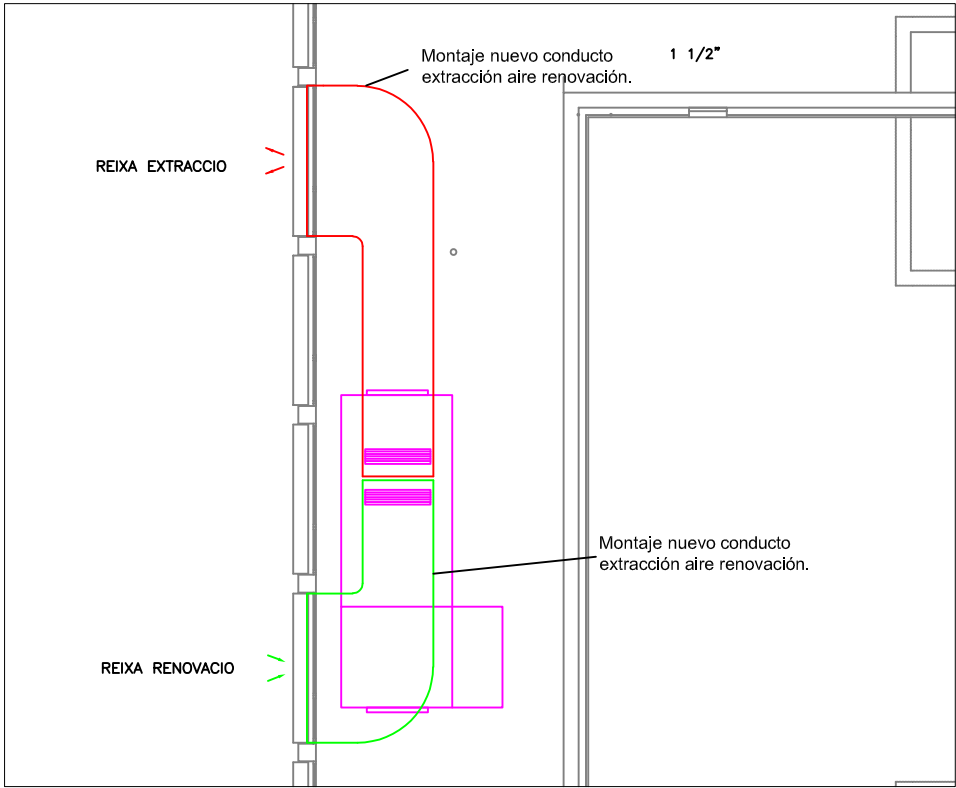
Nuevos conductos al exterior E 1:150
