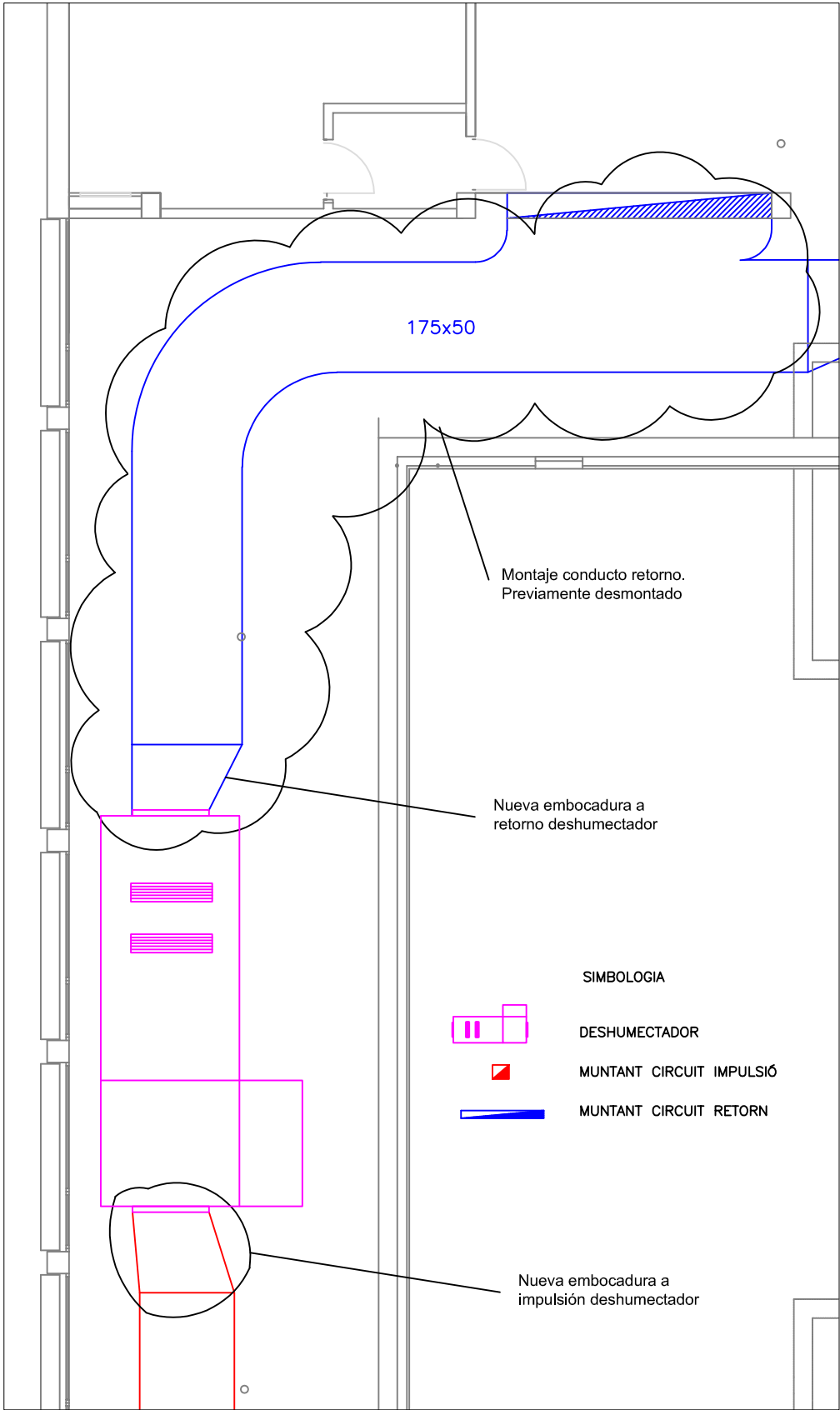
Adaptación conductos hacia la piscina
