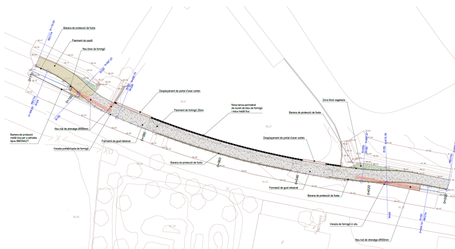
Figura 3. Planta general de l'actuació.
