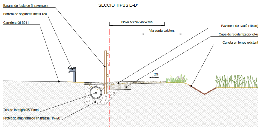
Figura 7. Secció tipus amb paviment de sauló.
