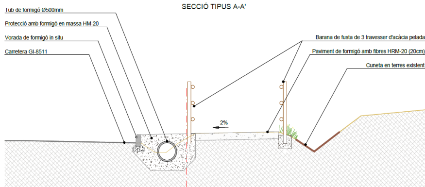
Figura 6. Secció tipus amb paviment de formigó.
