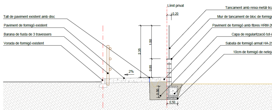
Figura 4. Secció tipus de la part central.
