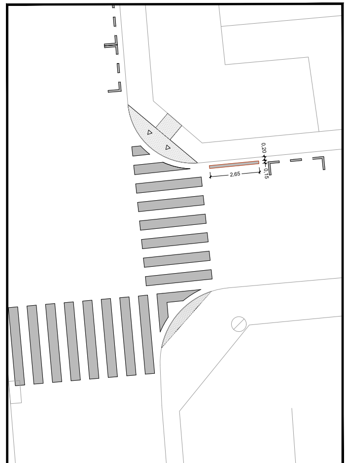
PROPOSTA ACTUACIÓ E.: 1/200
