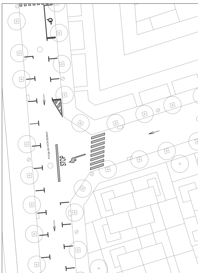
ESTAT ACTUAL E.: 1/200
