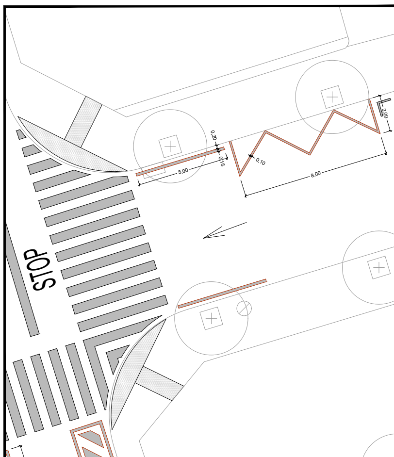
PROPOSTA ACTUACIÓ E.: 1/200
