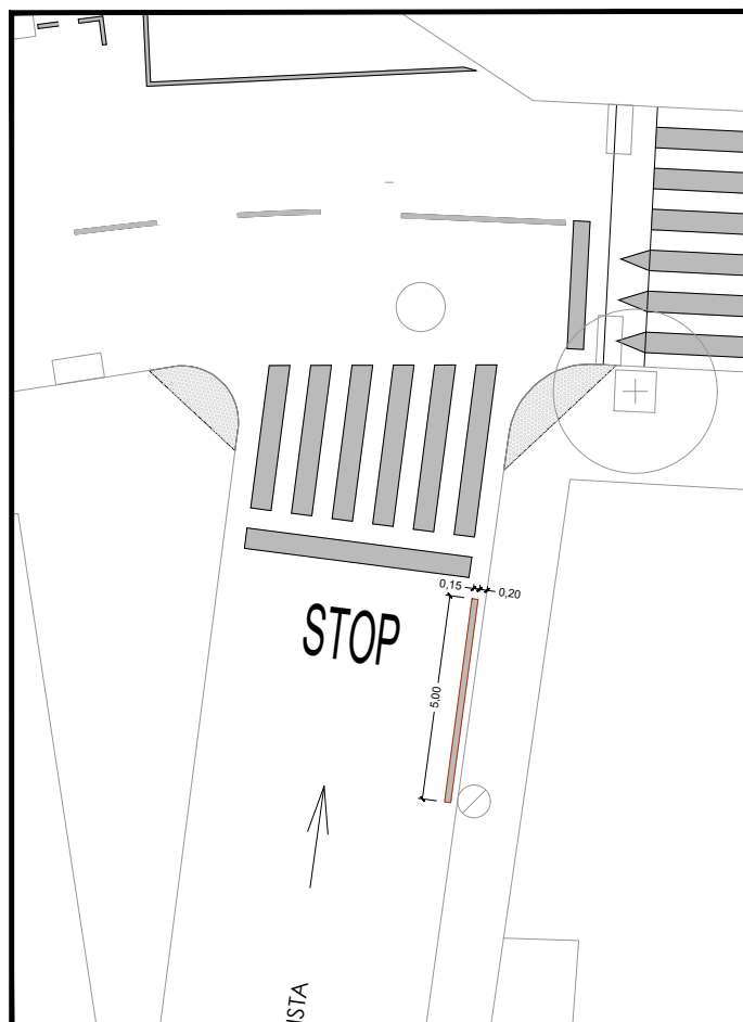
PROPOSTA ACTUACIÓ E.: 1/200
