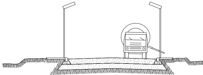
⑦ BASE GRANULAR FORMIGONAT VORERES i ESCOSELLS D ' ARBRES INSTAL·LACIË ENLLUMENAT
