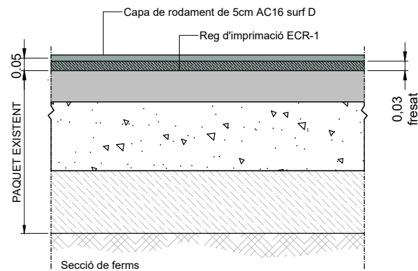
DETALL PAVIMENT D'AGLOMERAT ASFÀLTIC
