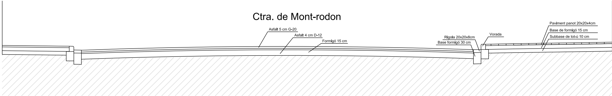
SECCIÓ ESTAT ACTUAL TIPUS
