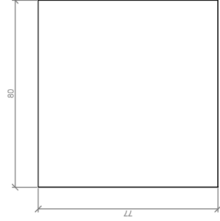
PERFIL / PROFIL VIEW ESCALA / SCALE 1/15
