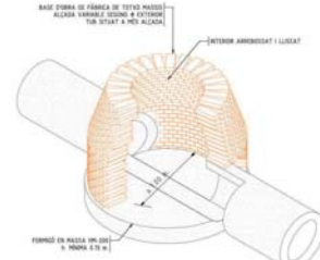
DETALL FORMACIÓ POU PETIT AMB CORA DE FÀBRICA
