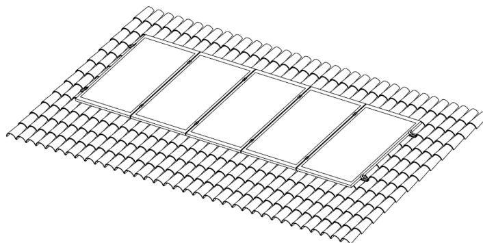
Fig. 6.2. Sistema de subjecció coplanar Aplisun.
