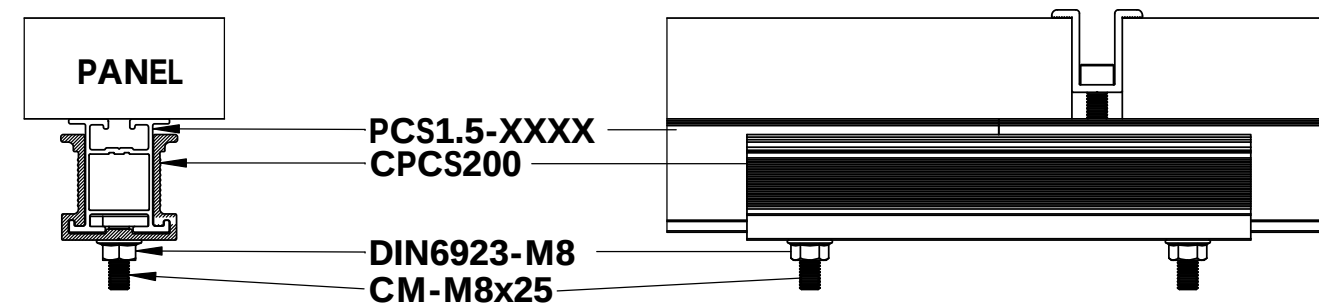
SECCIÓN D-D ESCALA 1:50
