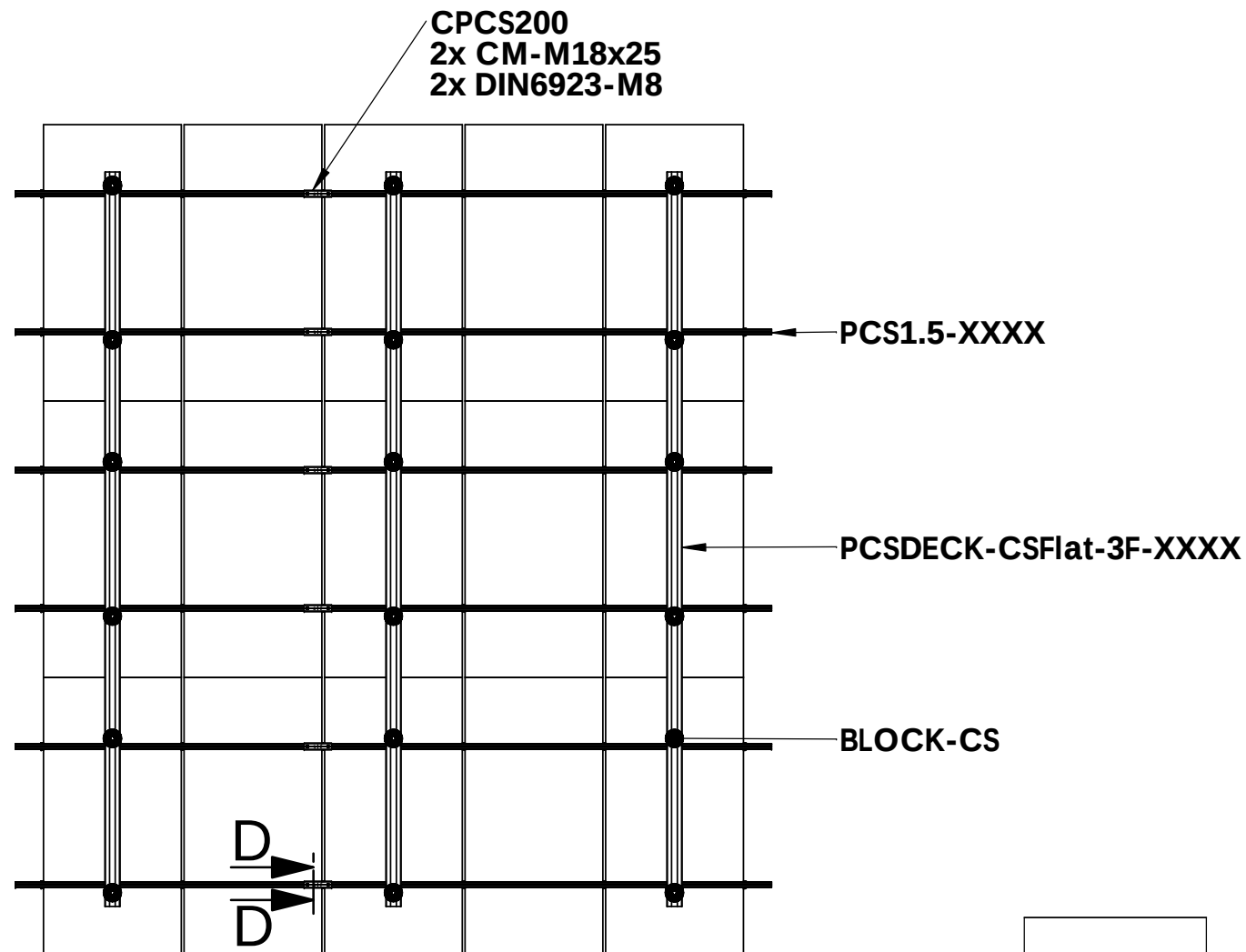
VISTA INFERIOR ESCALA 1:50
