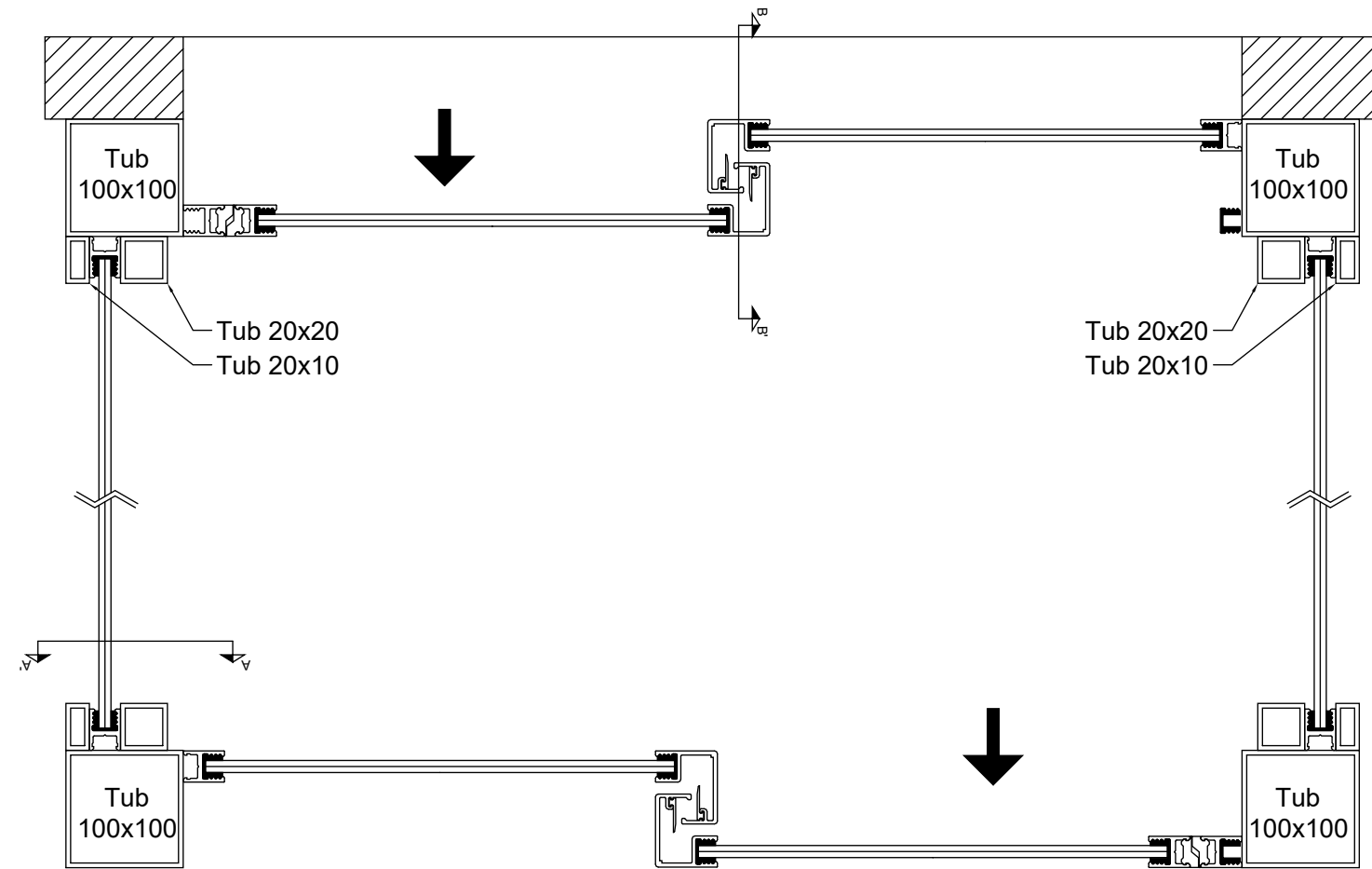
4 ACTUACIÓ 3 - DETALL PLANTA 03.3 1 : 30
