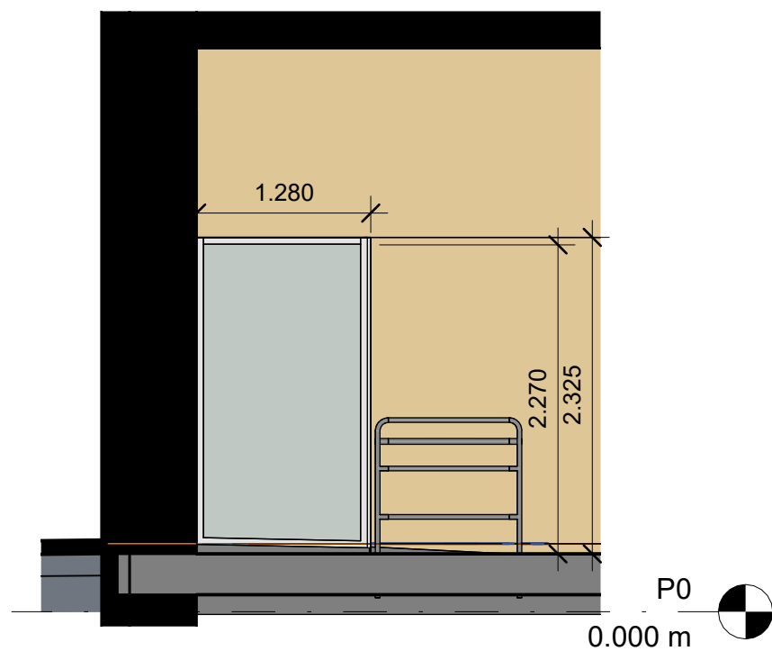
2 SECCIÓ LATERAL ACTUACIÓ 03 03.4 1 : 50
