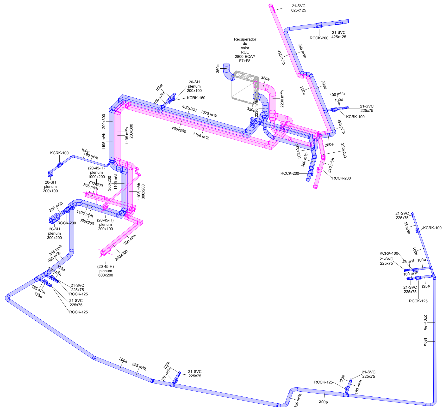
2 ISOMÈTRIC VENTILACIÓ 5.06/08
