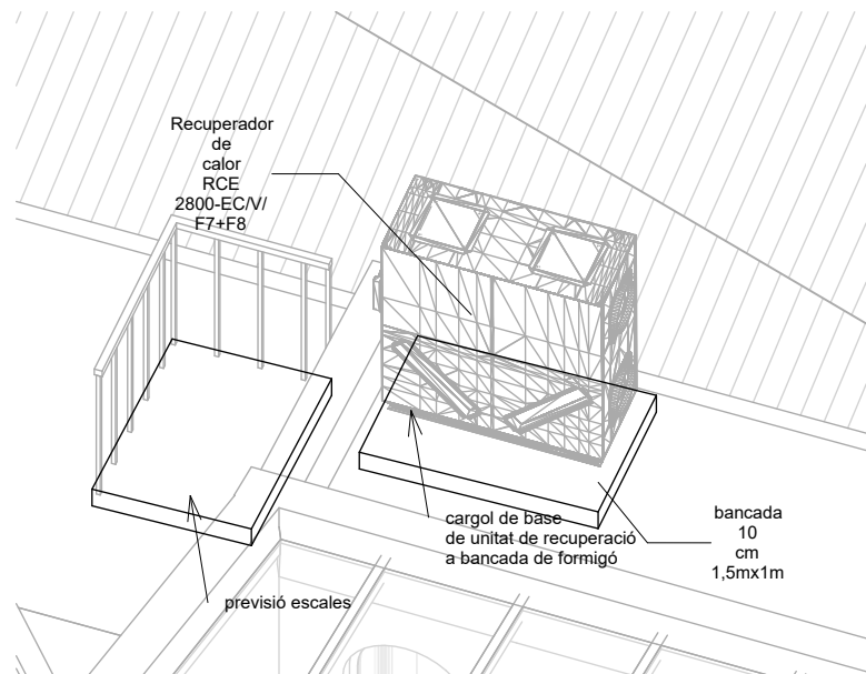
2 DETALL RECUPERADOR 2 5.06/06
