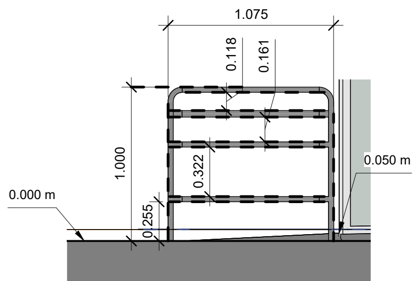
1 ALÇAT ACTUACIÓ 03 - BARANA 03.4 1 : 25
