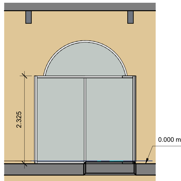
2 SECCIÓ LONGITUDINAL ACTUACIÓ 03 03.2 1 : 50
