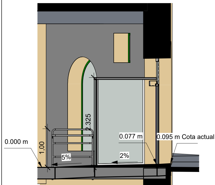
5 SECCIÓ ACTUACIÓ 03 03.2 1 : 50
