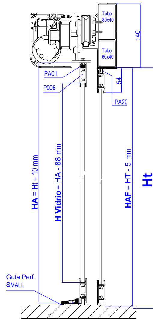
6 ACTUACIÓ 3 - DETALL SECCIÓ B I ACCIONAMENT 03.3 1 : 5
