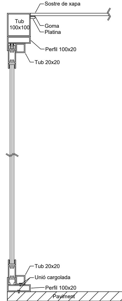
2 ACTUACIÓ 3 - DETALL SECCIÓ A PANELLS FIXES 03.3 1 : 5
