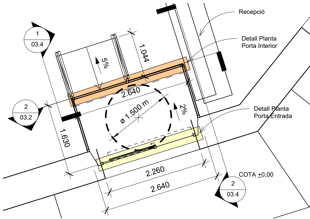
1 ACTUACIÓ 3 - SECCIONS 03.3 1 : 50
