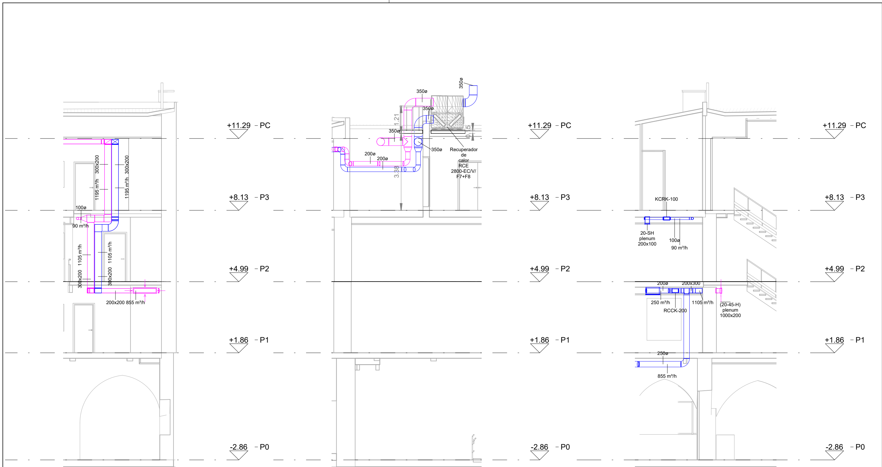
3 5.06/07 Secció 2 1 : 100
