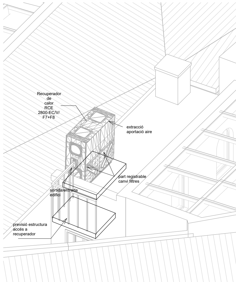
1 DETALL RECUPERADOR 1 5.06/06
