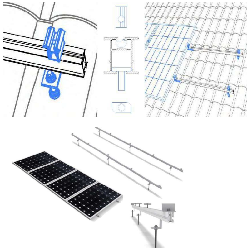
Detalls instal·lació de perfils i mòduls fotovoltaics.
