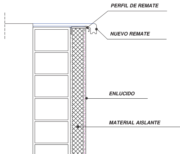
Antepecho cubierta*
