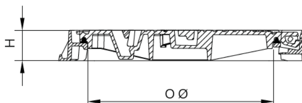
Secció
