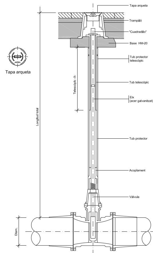
DETALL 030301 Válvula amb junta elàstica i eix telescòpic SENSE ESCALA
