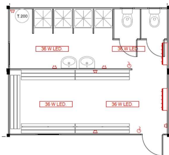
Planta
