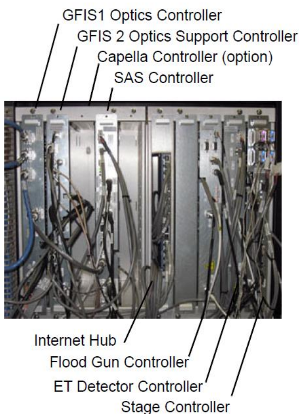
Fig: Vista del bastidor electrónico del microscopio nanofab Orion, incluido el controlador SAS.
