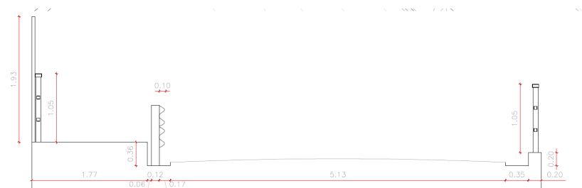
Figura 1. Secció pont estat actual
