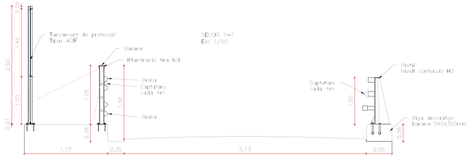
Figura 2. Secció pont proposada
