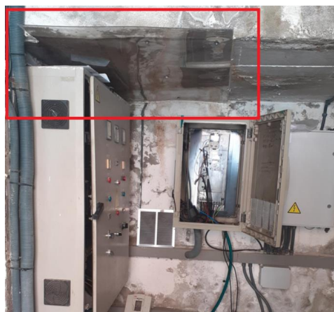
Imatges 2 i 3 – Estat de la instal·lació elèctrica de baixa tensió.
