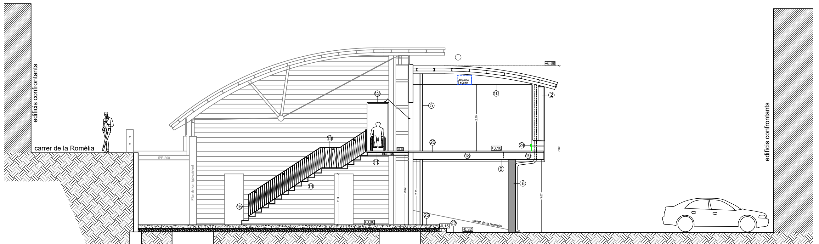
SECCIÓ LONGITUDINAL
