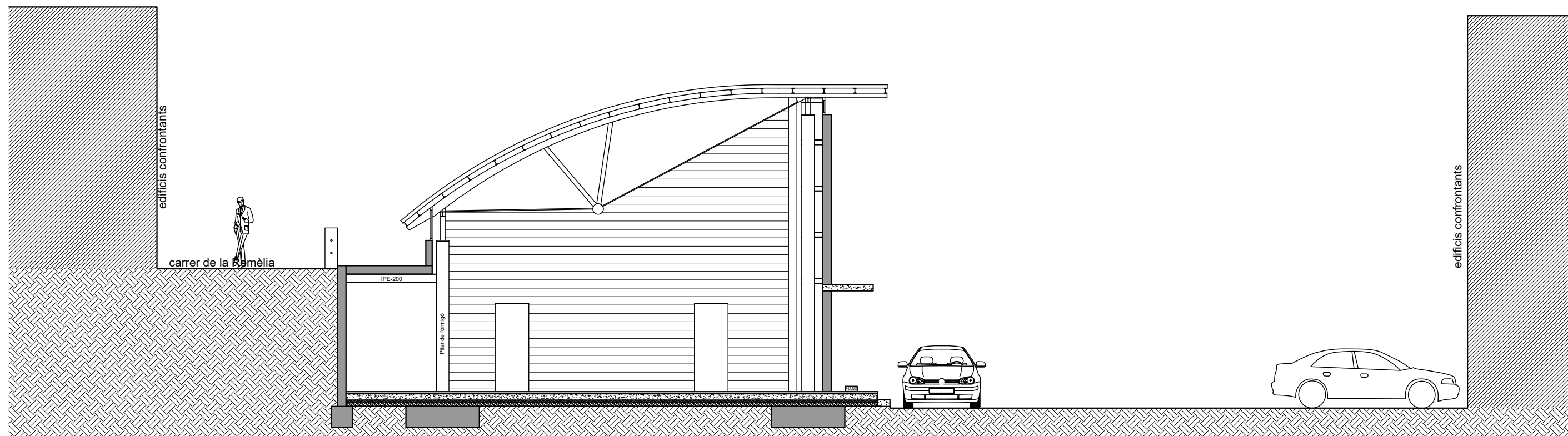
SECCIÓ
