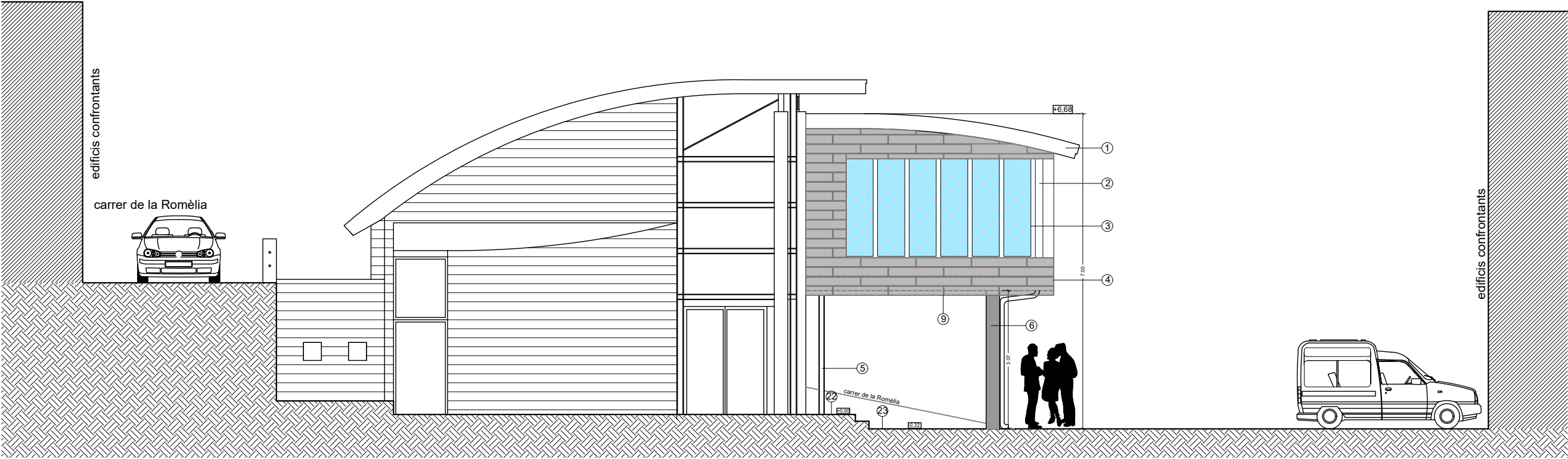
FAÇANA NORD
