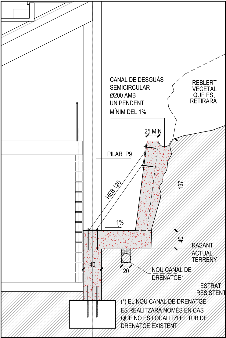
SECCIÓ A-A' - INTERVENCIÓ ESC 1:50
