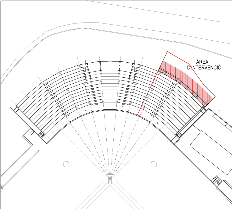
PLANTA REFERÈNCIA
