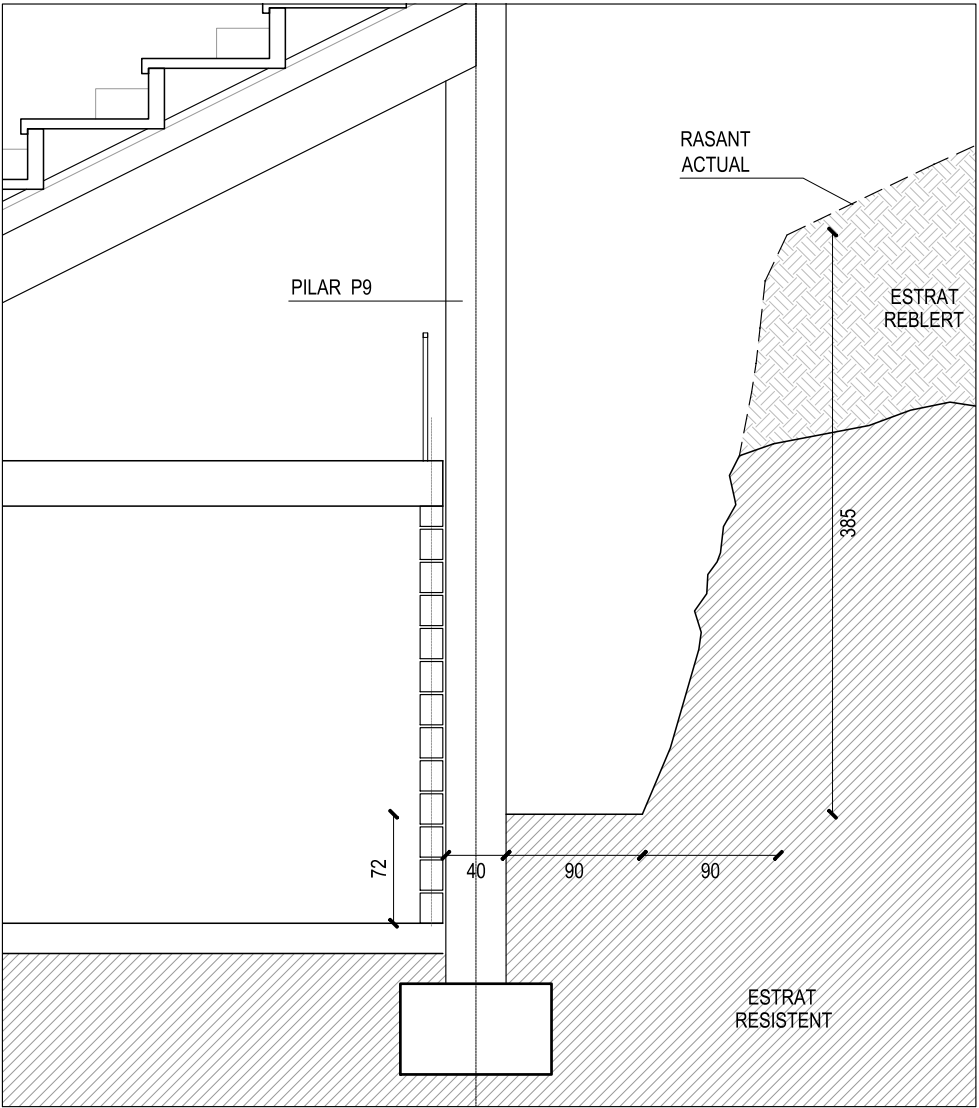
SECCIÓ A-A' - ESTAT ACTUAL ESC 1:50
