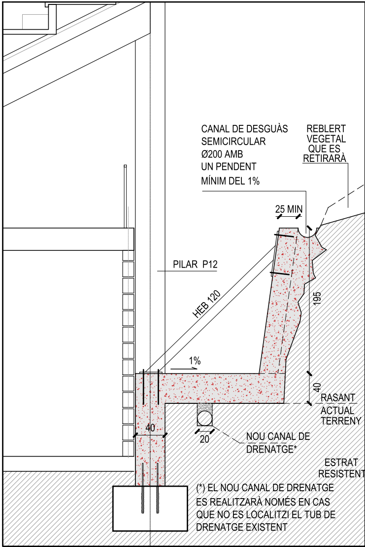
SECCIÓ C-C' - INTERVENCIÓ ESC 1:50
