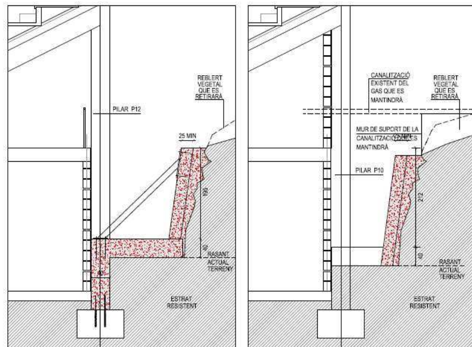
Figura 1.1. Secció del mur de contenció per la zona amb i sense sabata.
