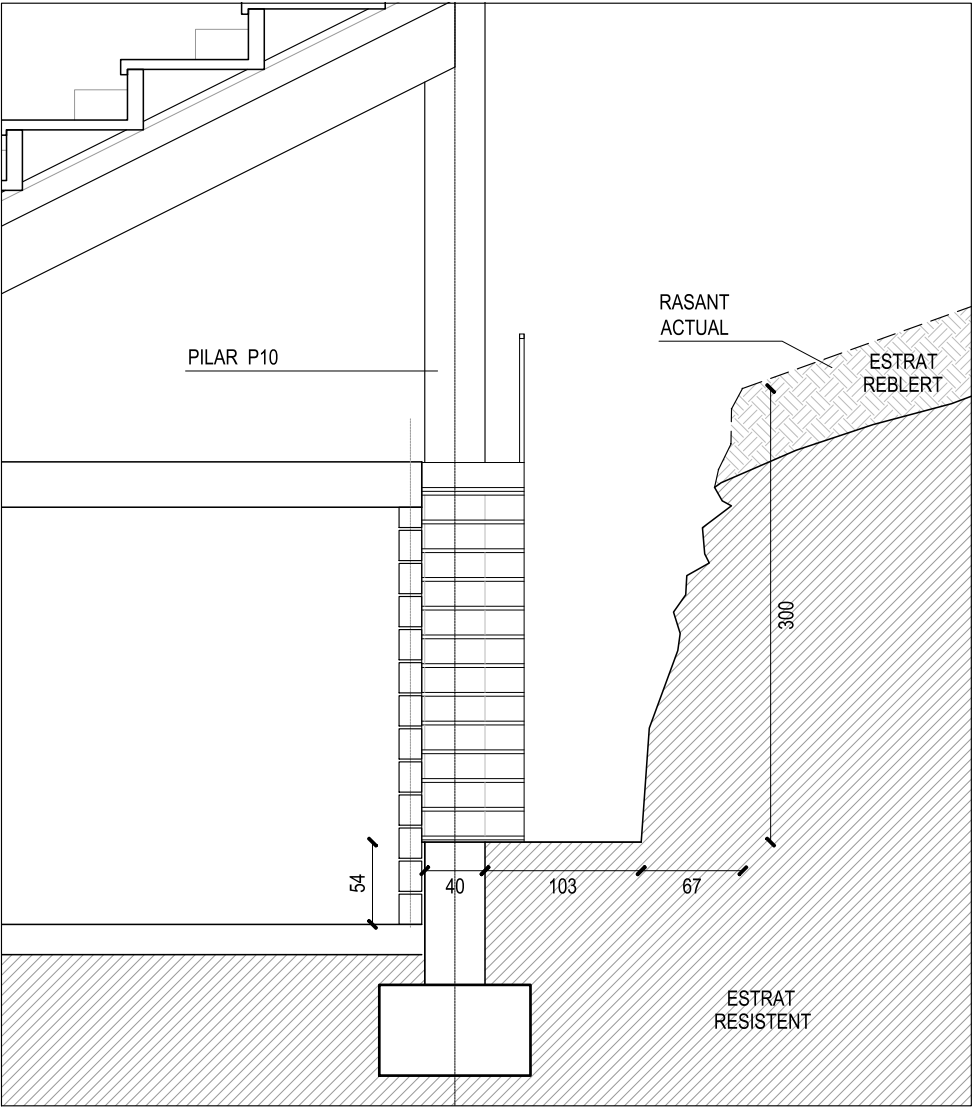
SECCIÓ B-B' - ESTAT ACTUAL ESC 1:50
