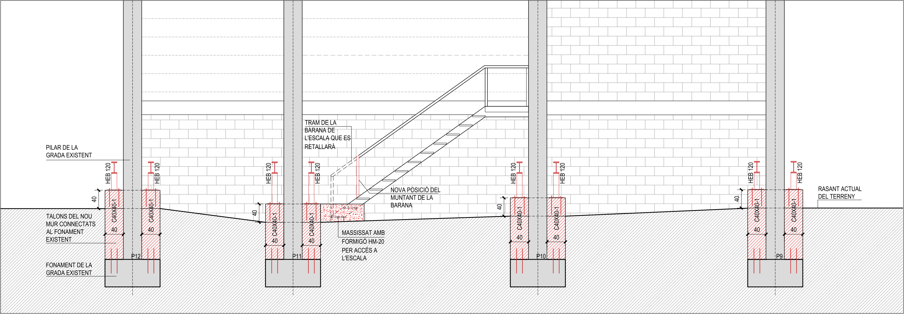
SECCIÓ E-E' - INTERVENCIÓ ESC 1:50
