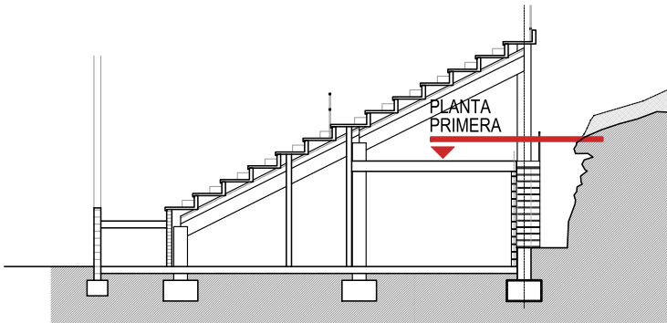
SECCIÓ REFERÈNCIA
