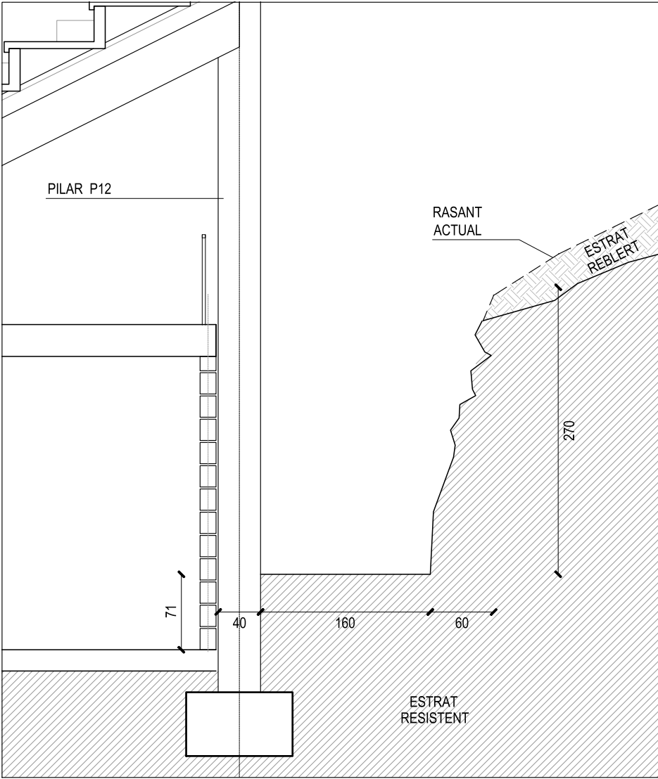
SECCIÓ C-C' - ESTAT ACTUAL ESC 1:50
