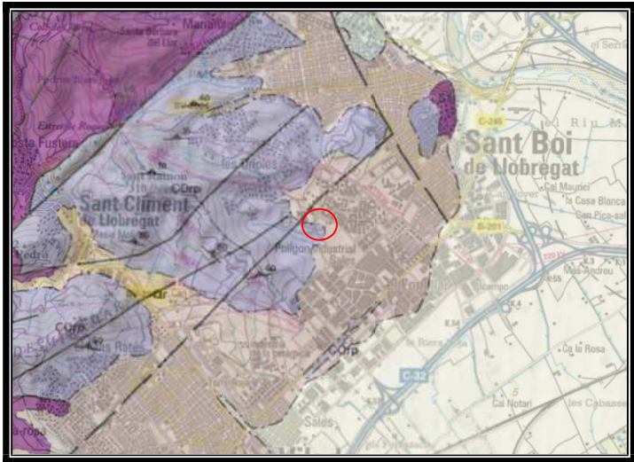
Mapa geològic de la zona d'estudi: en tons grisos els materials quaternaris; en color lila i morat les pissarres d'edat paleozoica.
