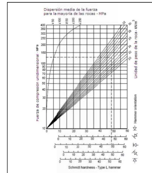
Àbac de correlacions de la resistència a la compressió simple
