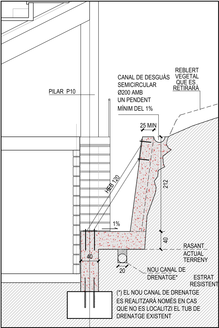
SECCIÓ B-B' - INTERVENCIÓ ESC 1:50
