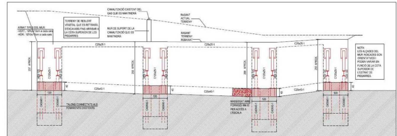
Figura 1.3. Alçat del mur de contenció mirant cap al talús de pissarres.
