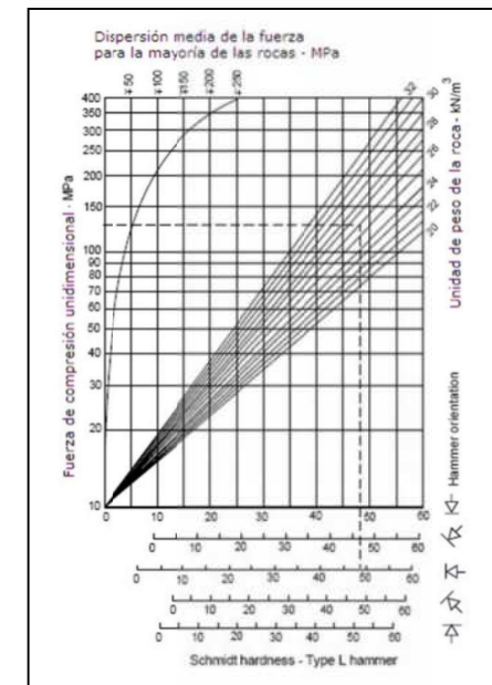
Assaig amb martell de Schmidt (escleròmetre).
