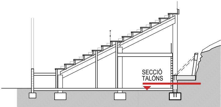
SECCIÓ REFERÈNCIA
