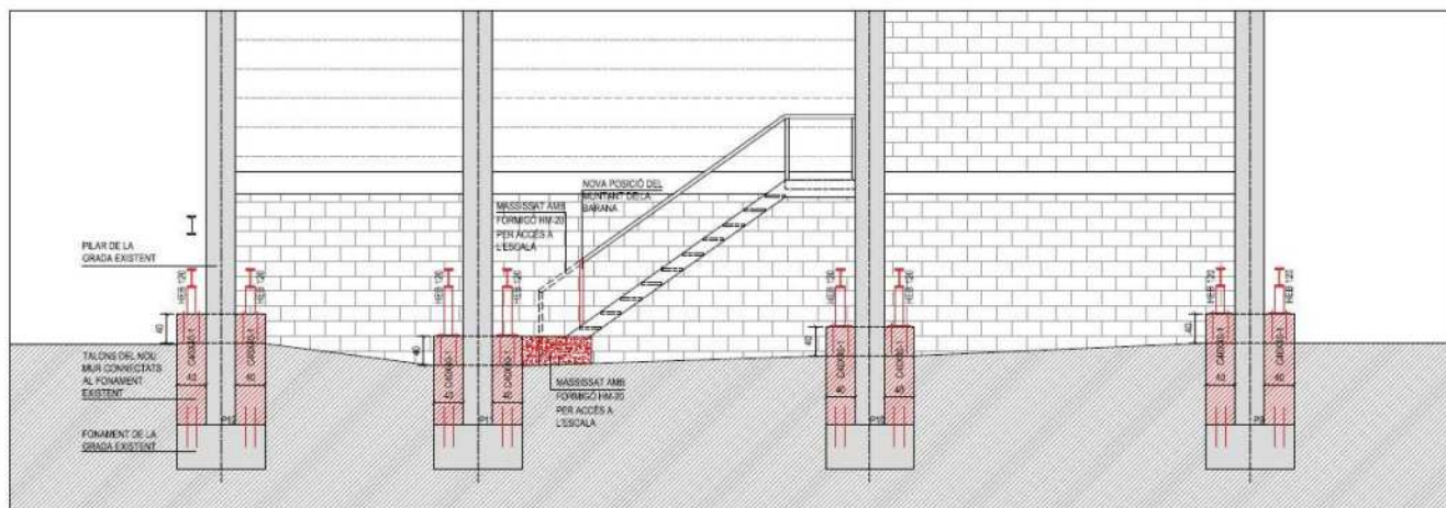
Figura 1.2. Alçat del nou mur de contenció mirant cap a les grades.
