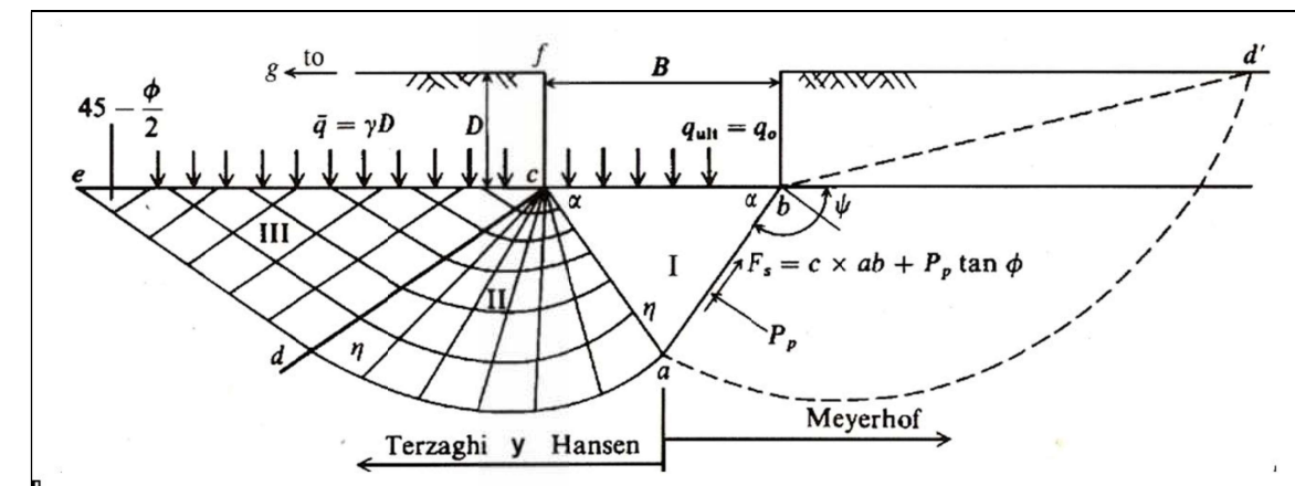
Distribució d'esforços en les principals formulacions
