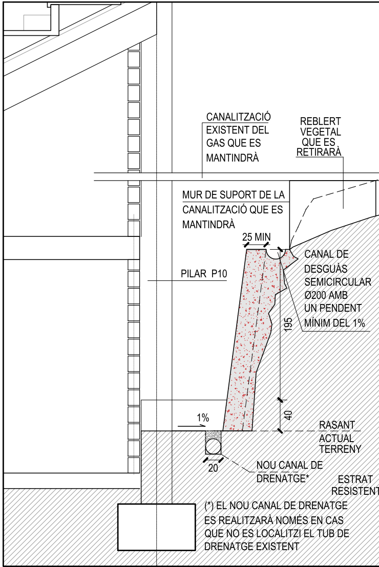
SECCIÓ D-D' - INTERVENCIÓ ESC 1:50
