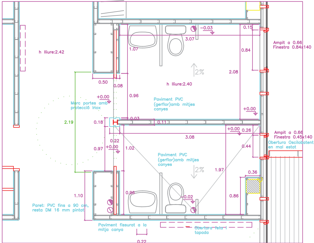
PLANTA SEGONA – LAVABOS ALA INTERIOR
