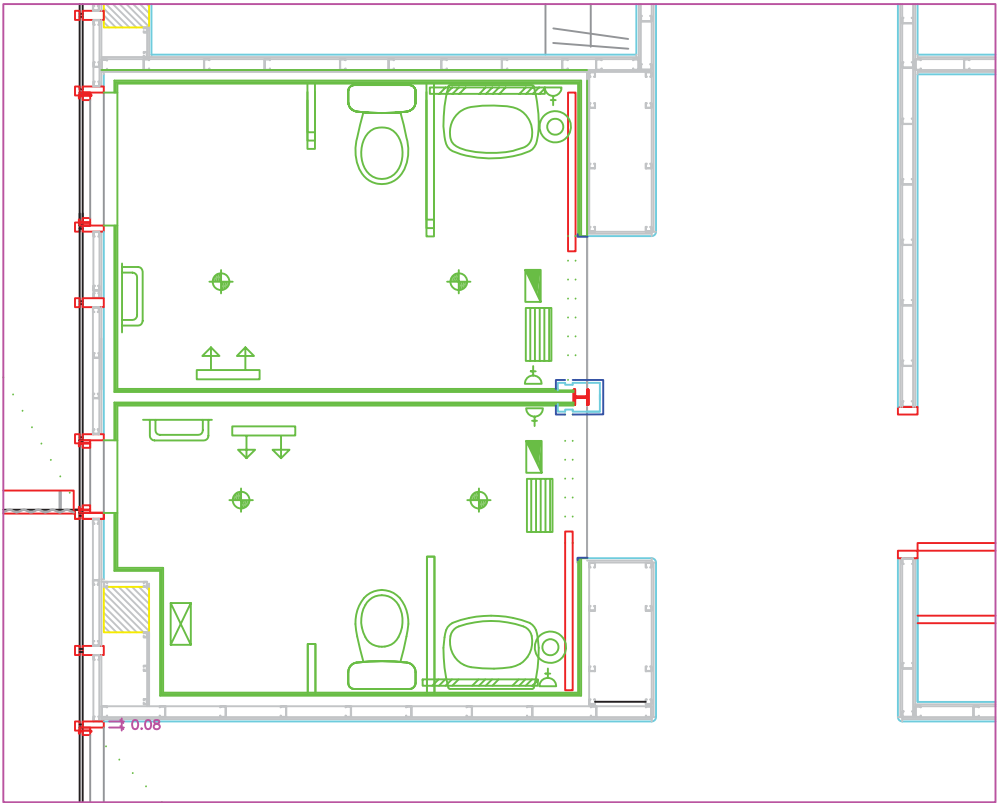
PLANTA PRIMERA - LAVABOS ALA VIAL
