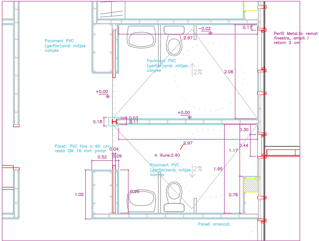
PLANTA PRIMERA – LAVABOS ALA INTERIOR
