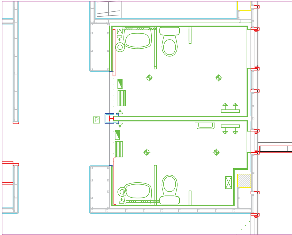
PLANTA PRIMERA - LAVABOS ALA INTERIOR
