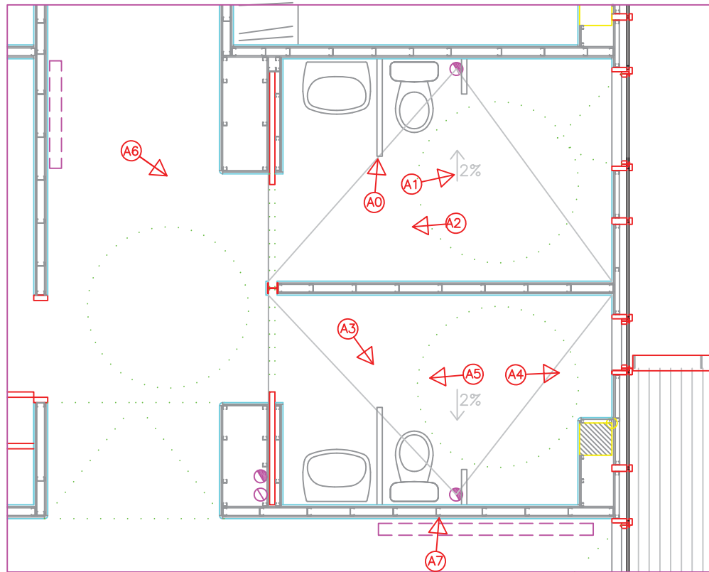
PLANTA SEGONA - LAVABOS ALA INTERIOR
