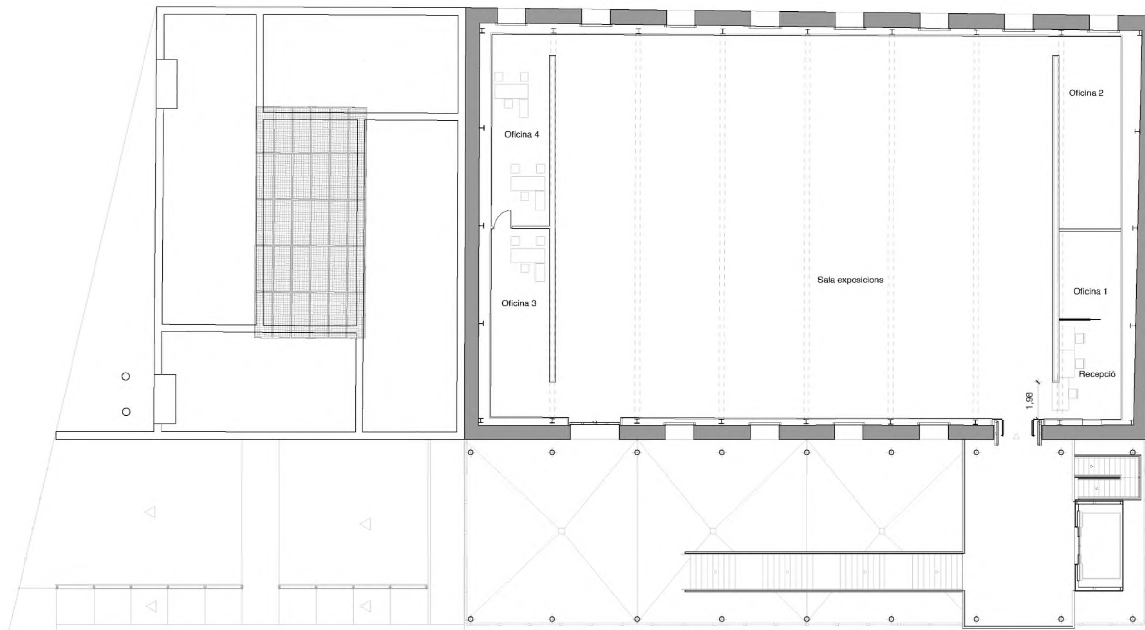
Planta primera
