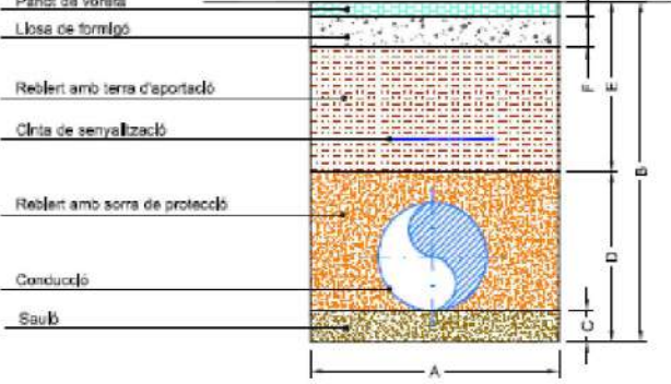
RASA TIPUS EN VORERA
