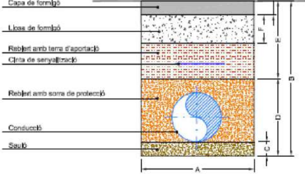
RASA TIPUS EN FORMIGÓ
