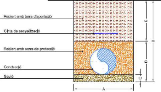
RASA TIPUS EN TERRA
