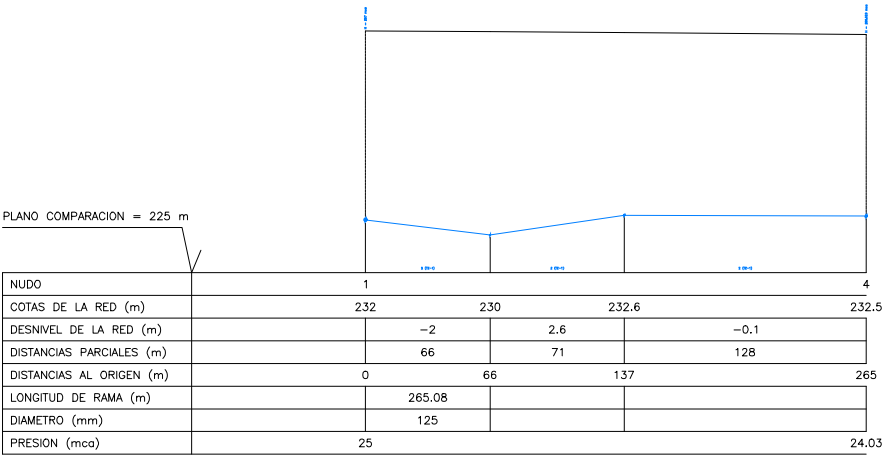
PERFIL LONGITUDINAL 1-4
