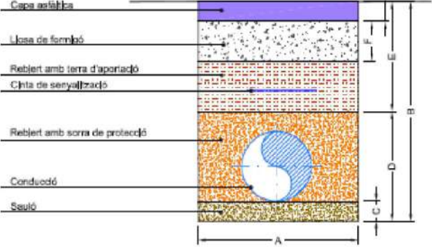
RASA TIPUS EN ASFALT
