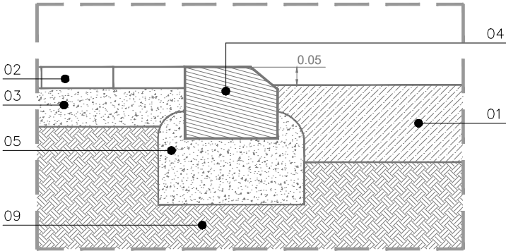
SECCIÓ TROBADA VORERA FORMIGÓ AMB SAULÓ PATI E 1/15
