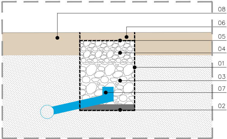
SECCIÓ ACABAT PATI I POU DE DRENATGE E 1/25
