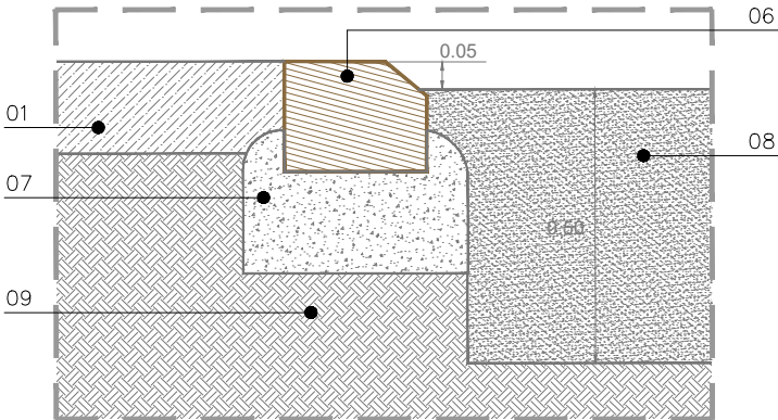
SECCIÓ TROBADA PAVIMENT SAULÓ AMB SORRAL E 1/15
