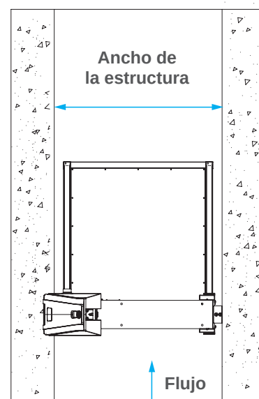
Vista de planta
