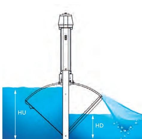
Niveles hídricos aguas arriba y agua abajo
