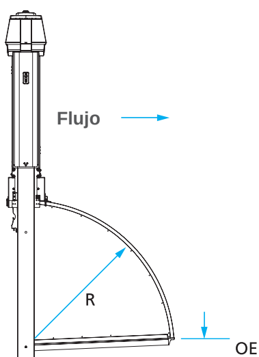
Vista lateral - compuerta completamente abierta
