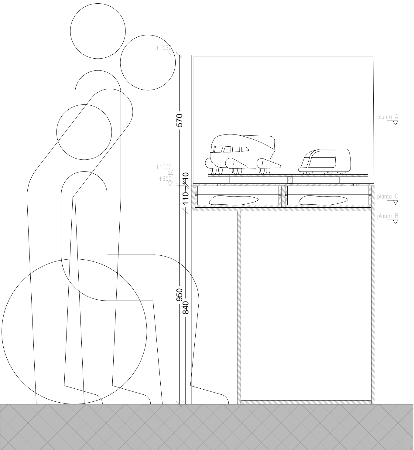
SECCIÓN
