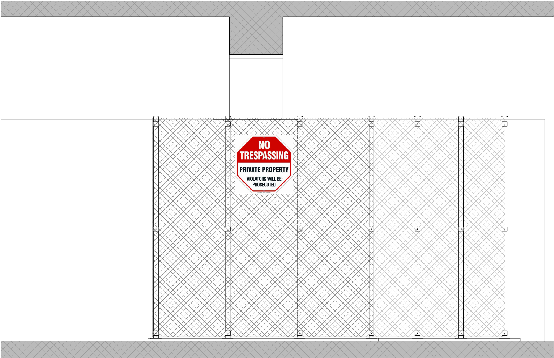
ALZADO 1/25
