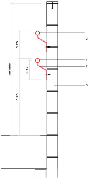
SECCIÓ DE LA BARANA E: 1/20
