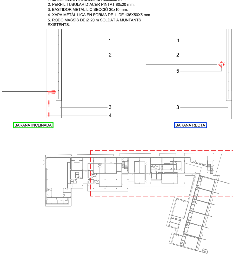
SECCIÓ EXTERIOR DE LA BARANA E: 1/25
