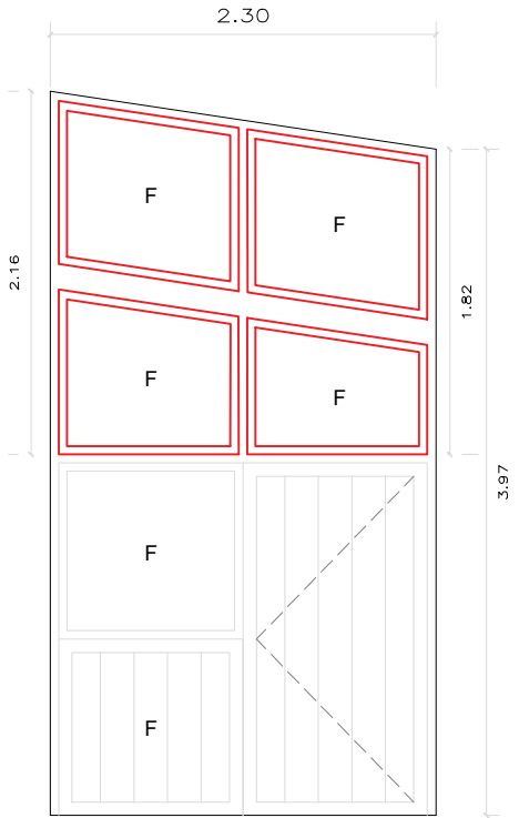
DETALL FUSTERIA GIMNÀS E: 1/50
