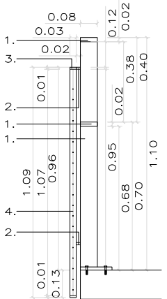
SECCIÓ DE LA BARANA E: 1/25
