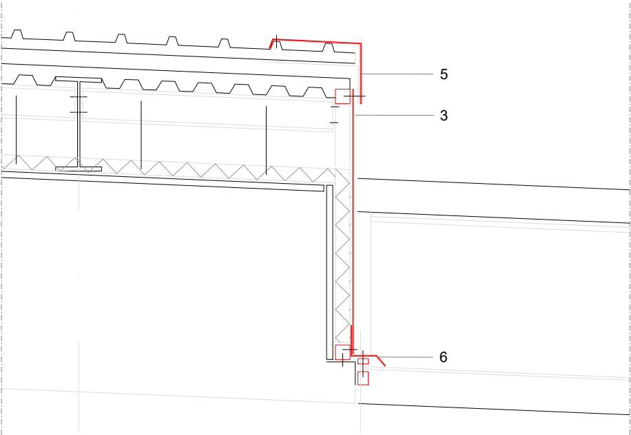
SECCIÓ DETALL LLUERNARI E: 1/25
