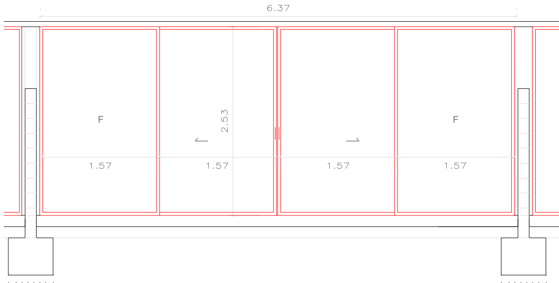
DETALL FUSTERIA AULES INFANTILS E: 1/50
