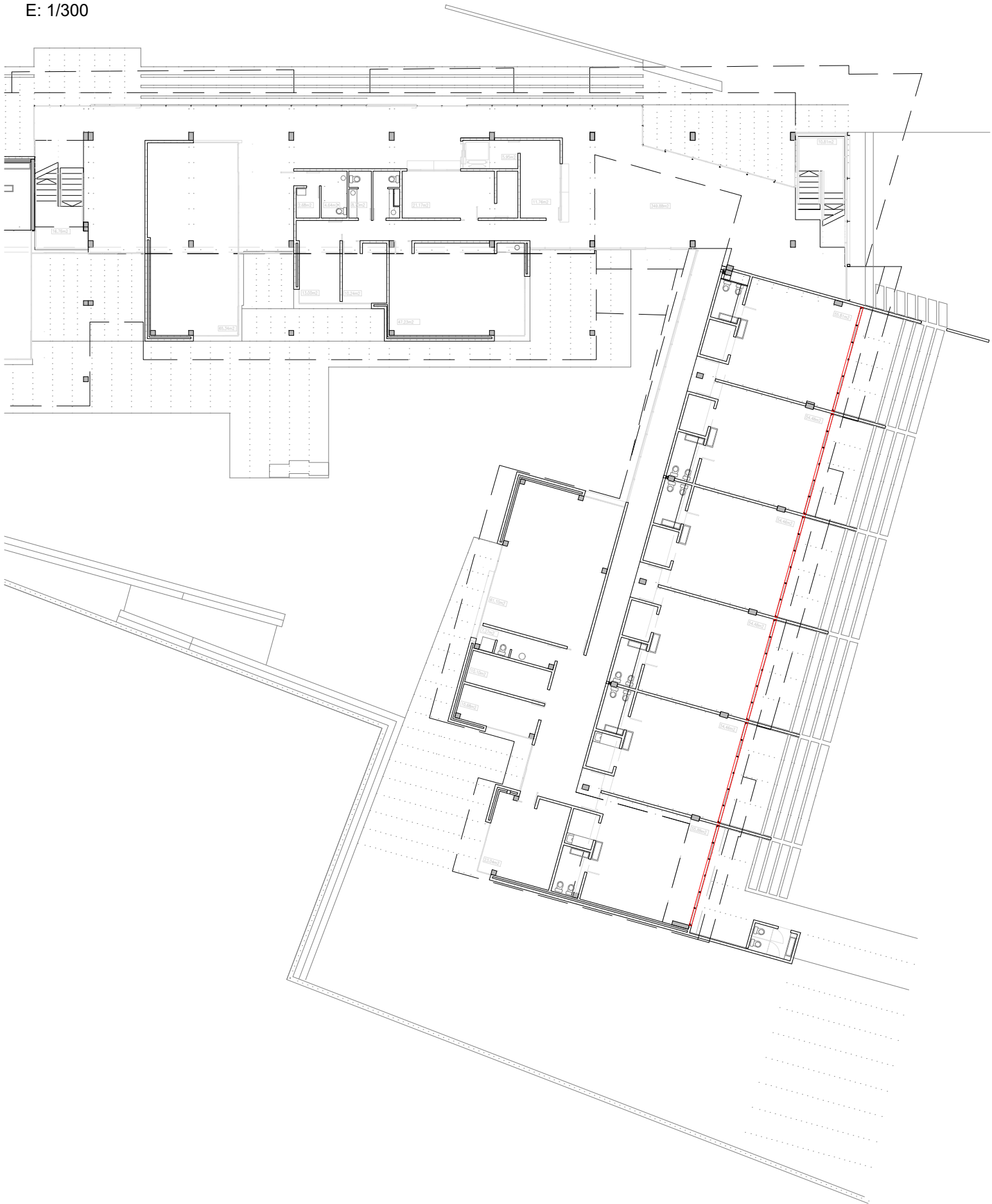
PLANTA BAIXA E: 1/300
