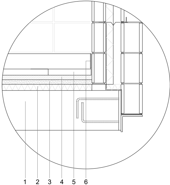
DETALL PAVIMENT EXISTENT E: 1/15
