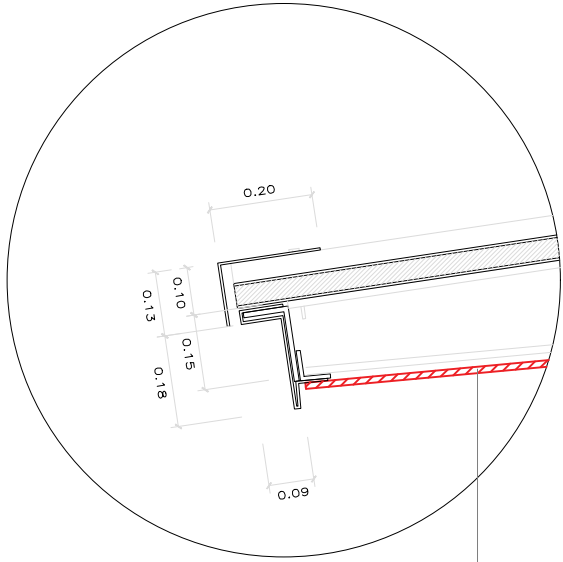
CEL RAS PROPOSTA D1 E: 1/15
