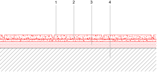
DETALL PAVIMENT DE FORMIGÓ
