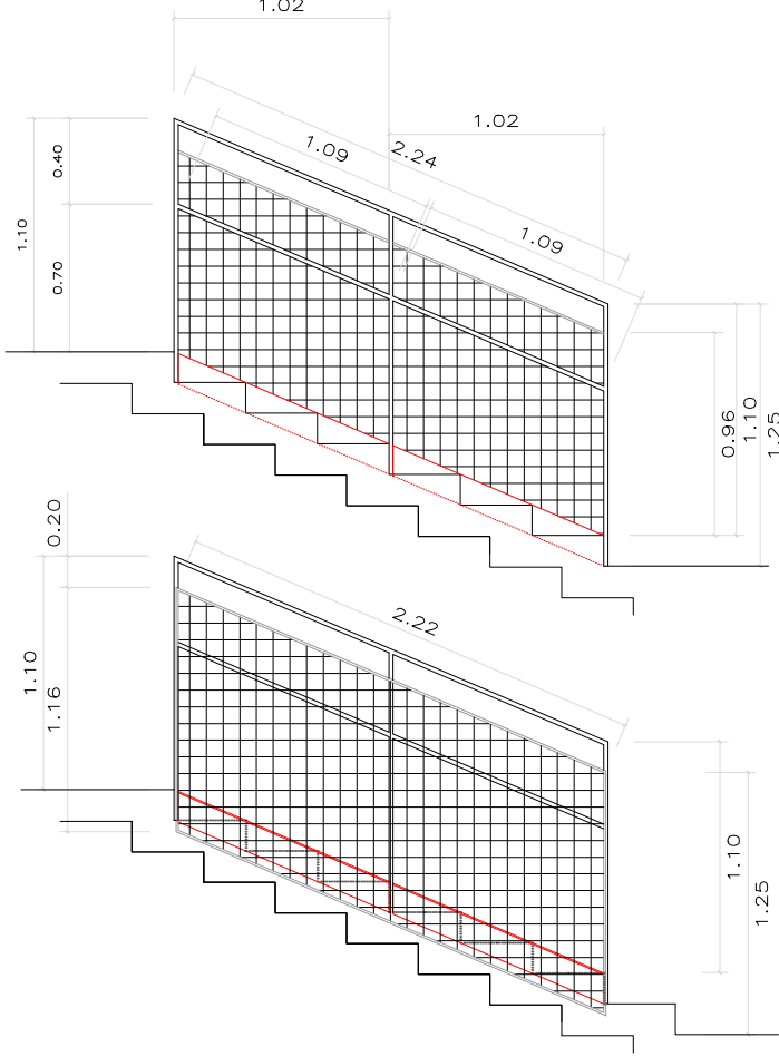
ALÇAT INTERIOR I EXTERIOR E: 1/40
