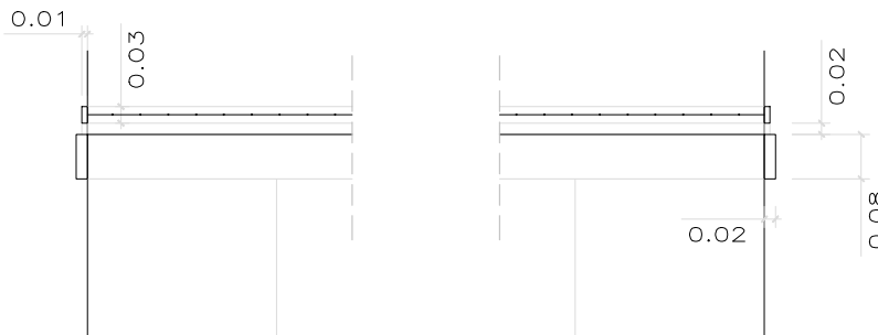
DETALL DE LA BARANA EN PLANTA E: 1/15
