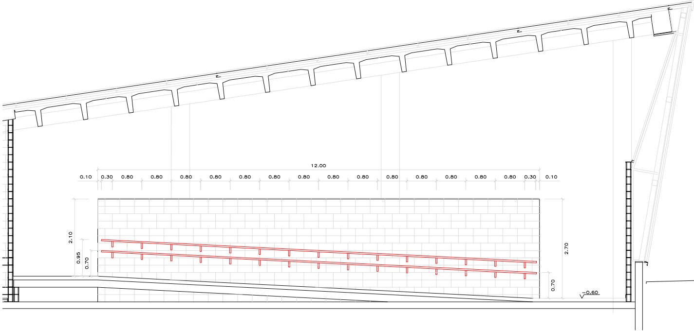
SECCIÓ DE LA BARANA E: 1/20
