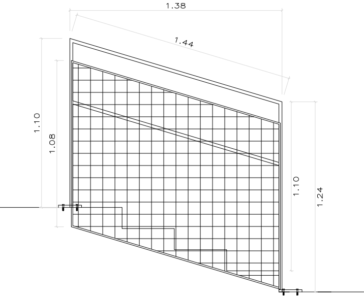
ALÇAT EXTERIOR E: 1/25
