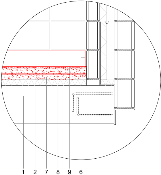
DETALL PAVIMENT PROPOSTA E: 1/15
