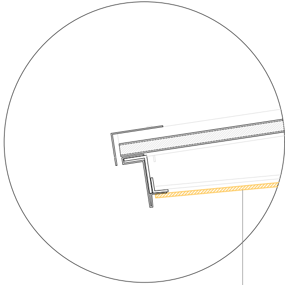
CEL RAS EXISTENT D1 E: 1/15
