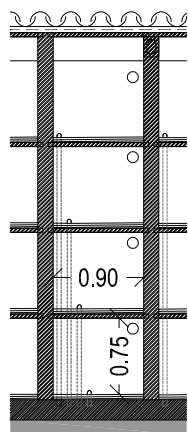
SECCIÓ TRANSVERSAL
