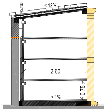
SECCIÓ LONGITUDINAL
