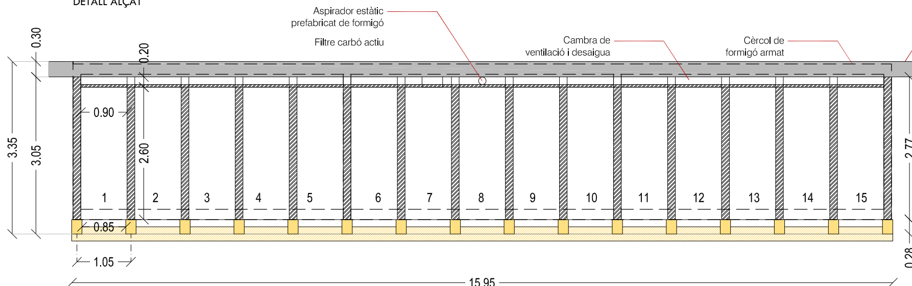
PLANTA
