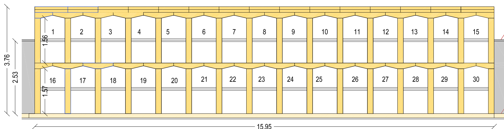
DETALL ALÇAT
