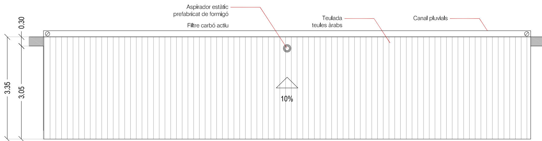
PLANTA COBERTA
