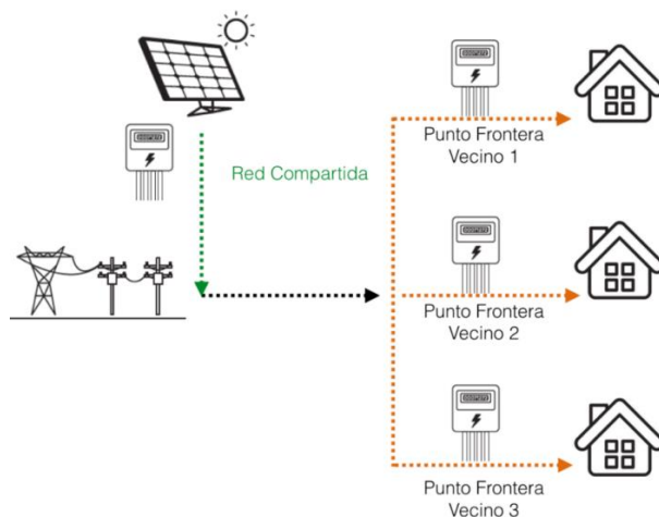
Figura 3. Esquema de funcionamiento de una instalación fotovoltaica conectada de autoconsumo compartido.
