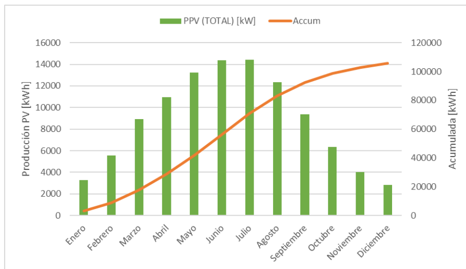
Figura 5. Producción mensual y anual de electricidad para la situación óptima y la integración real.
