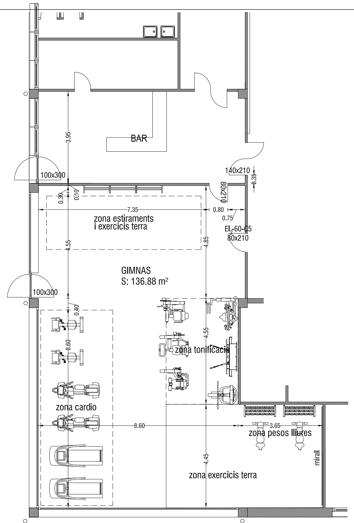
PLANTA DEFINITIVA DISTRIBUCIÓ I COTES
