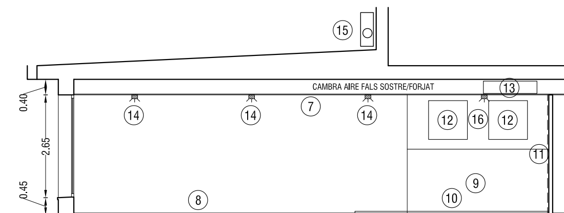
SECCIÓ B-B'
