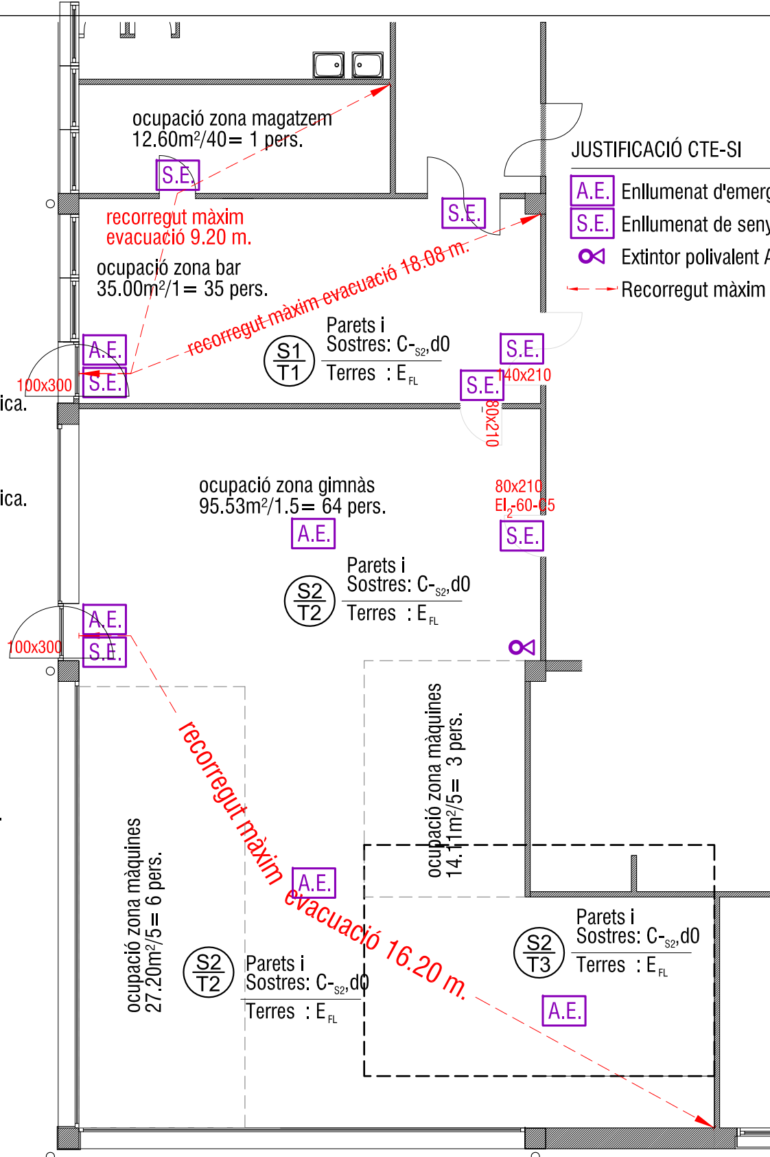
PLANTA DEFINITIVA JUSTIFICACIÓ CTE-SI
