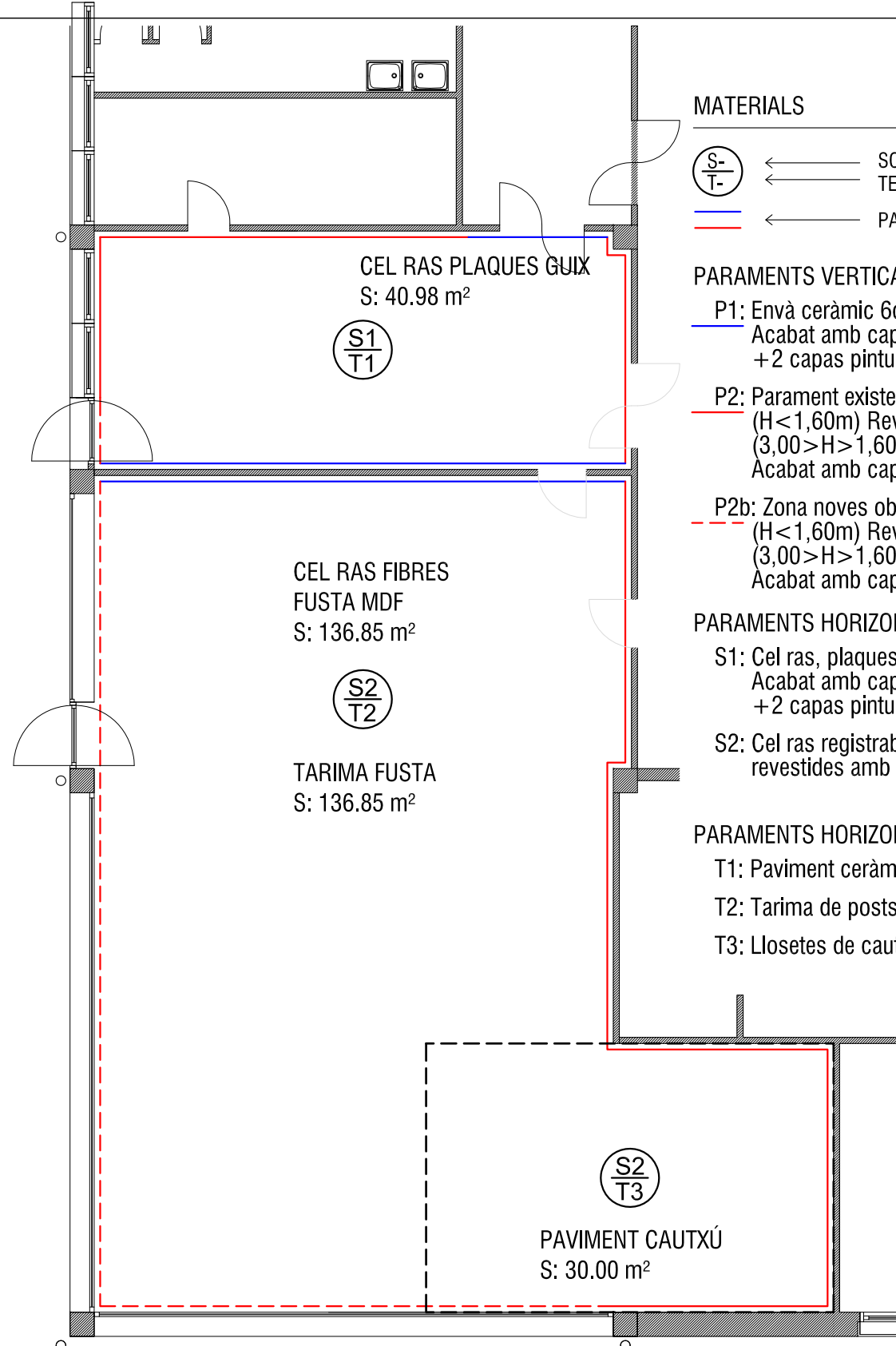
PLANTA DEFINITIVA PLÀNOL DE MATERIALS
