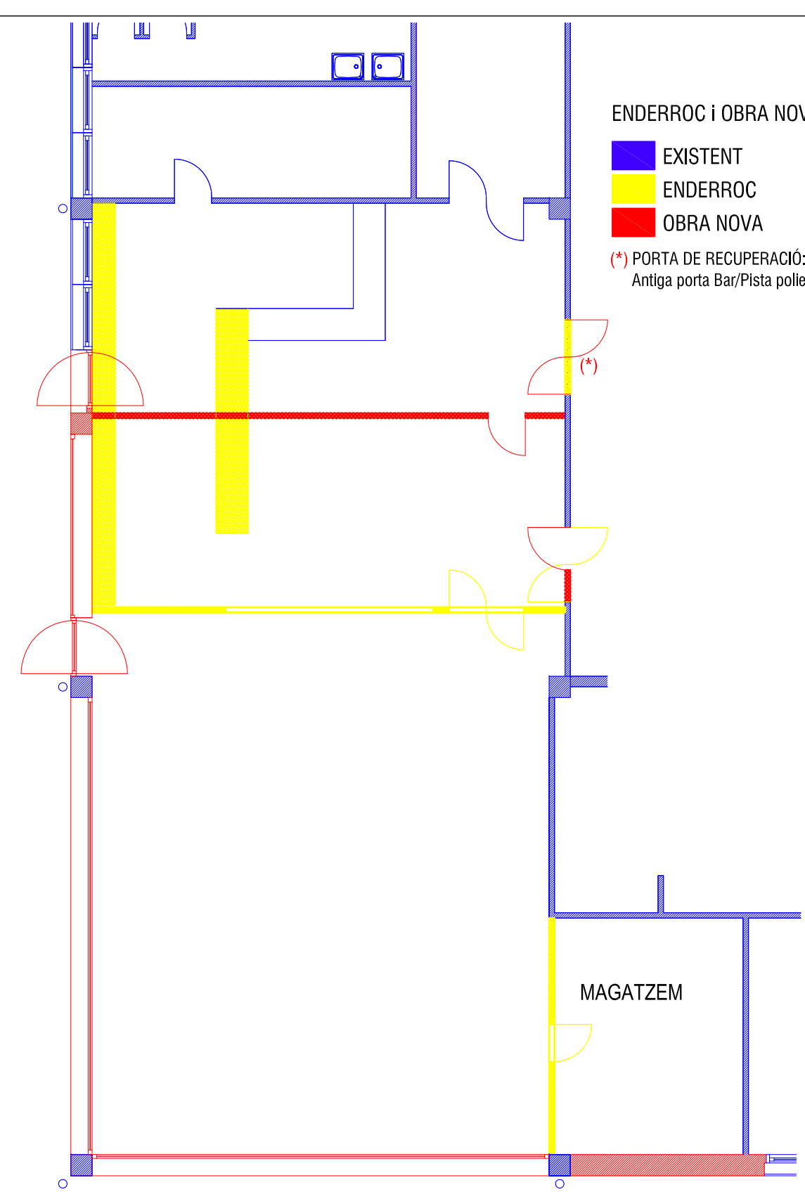
PLANTA ESTAT ACTUAL/PROPOSTA
